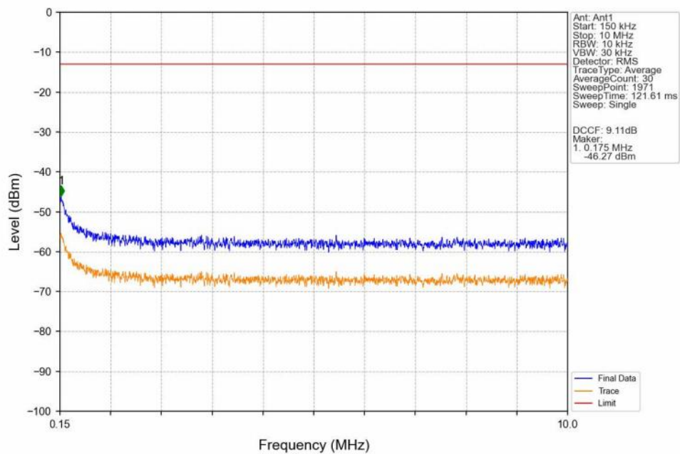
GSM850_GPRS_HCH_848.8MHz_1_TX_Slot_NTNV
