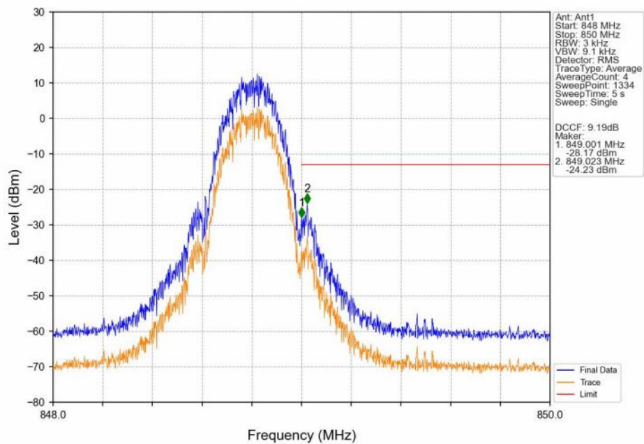
GSM850 EGPRS HCH 848.8MHz 1 TX Slot NTN
