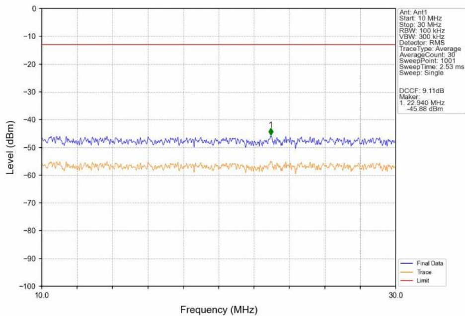
GSM850 GSM MCH 836.6MHz GSM NTN
