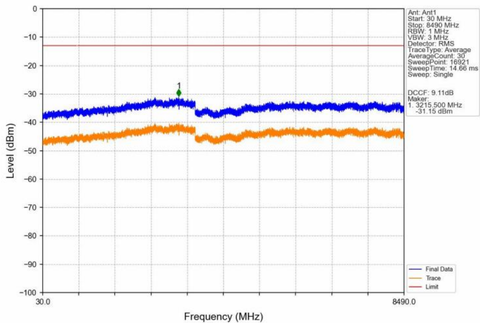
GSM850_GPRS_HCH_848.8MHz_1_TX_Slot_NTNV
