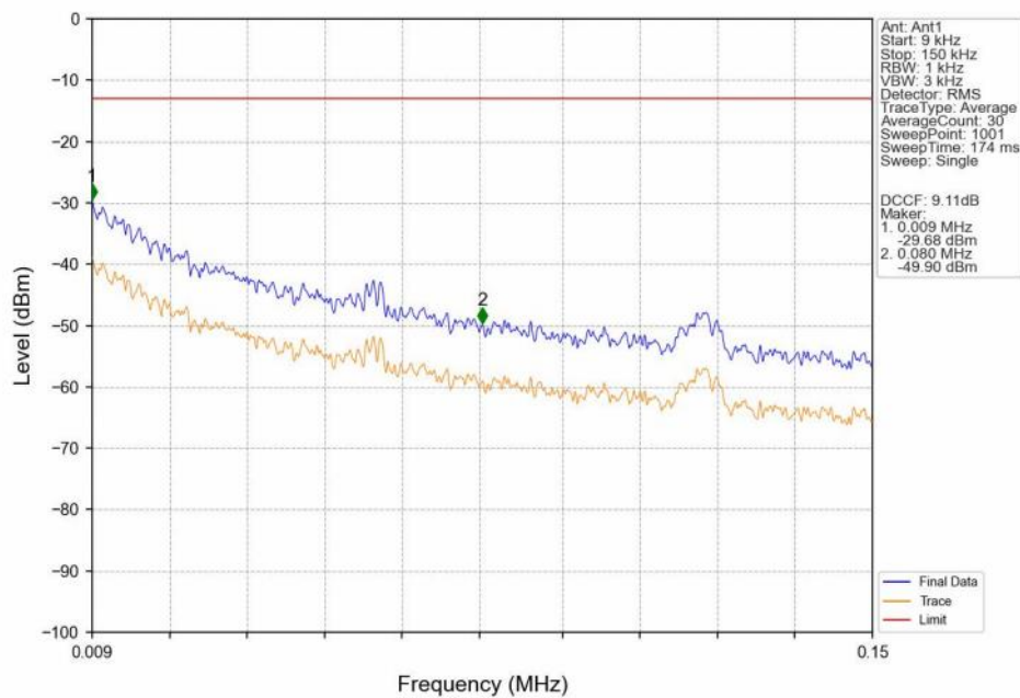
GSM850_GPRS_LCH_824.2MHz_1_TX_Slot_NTNV
