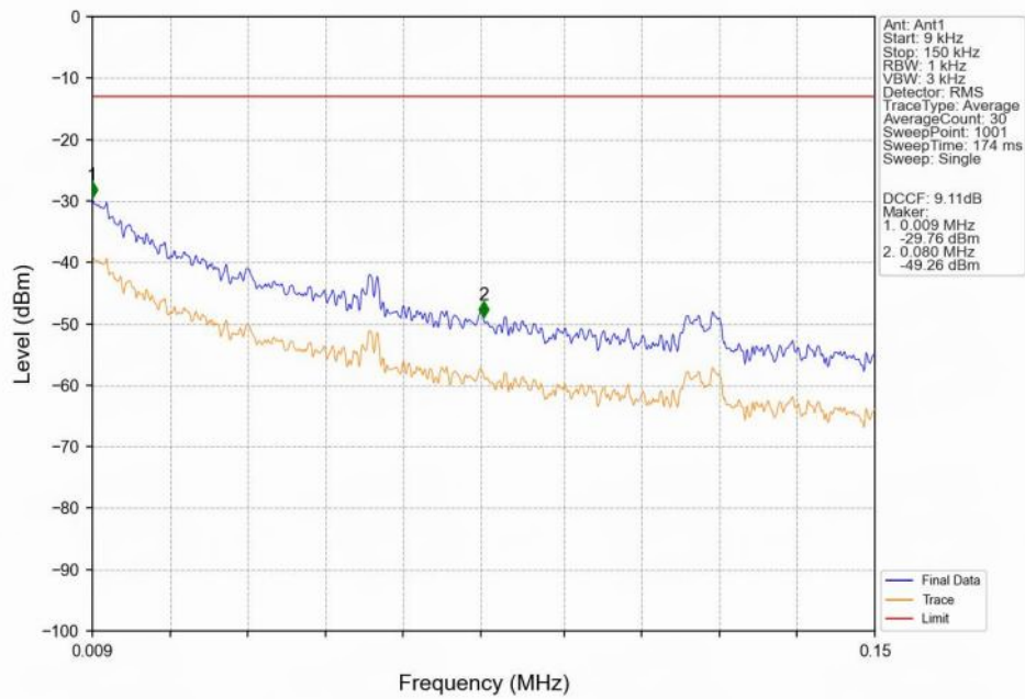
GSM850_GPRS_HCH_848.8MHz_1_TX_Slot_NTNV
