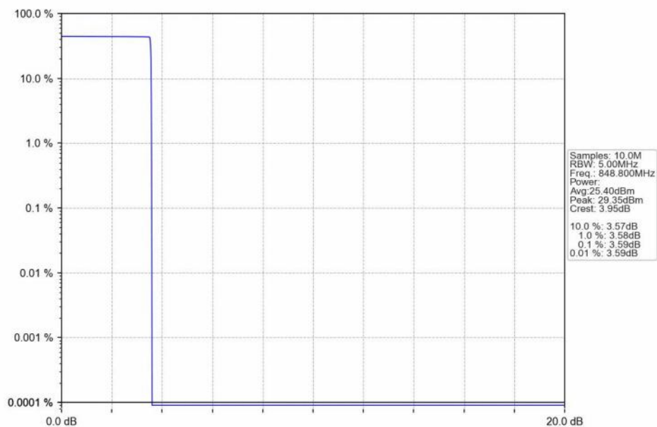
GSM850 GPRS HCH 848.8MHz 4 TX Slots NTV
