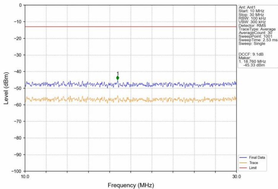
GSM850 GSM LCH 824.2MHz GSM NTNV
