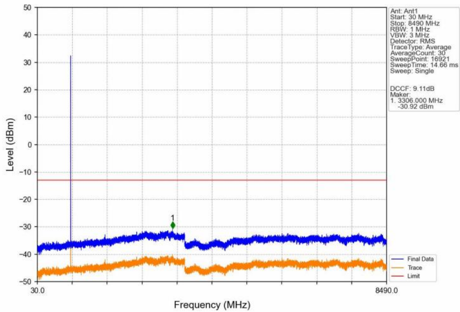
GSM850 GSM HCH 848.8MHz GSM NTN
