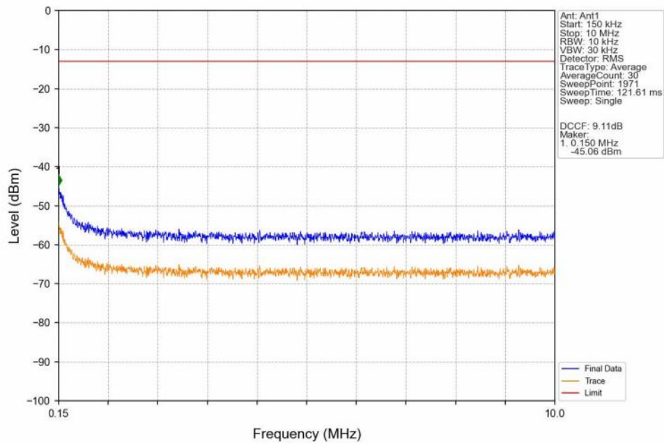
GSM850_GPRS_LCH_824.2MHz_1_TX_Slot_NTNV
