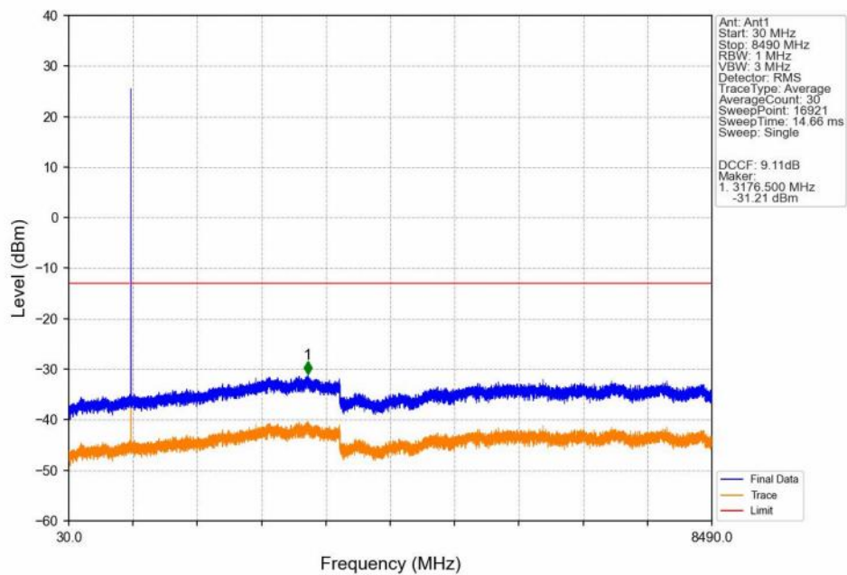
GSM850 GSM HCH 848.8MHz GSM NTNV
