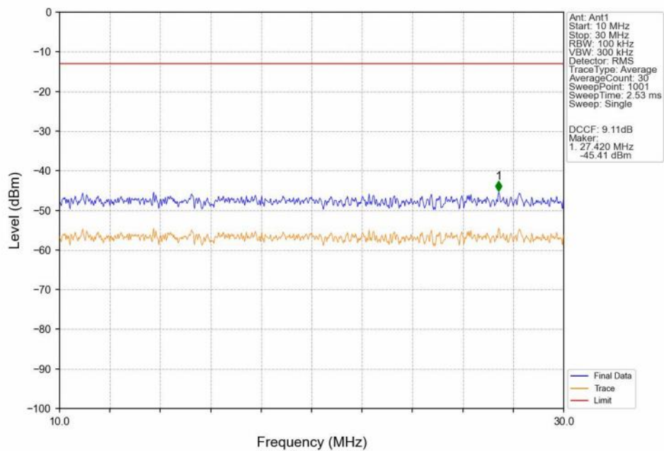
GSM850_GPRS_LCH_824.2MHz_1_TX_Slot_NTNV
