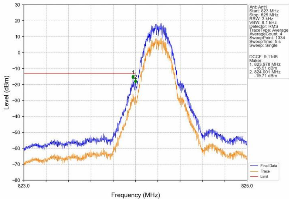
GSM850_GPRS_LCH_824.2MHz_1_TX_Slot_NTNV
