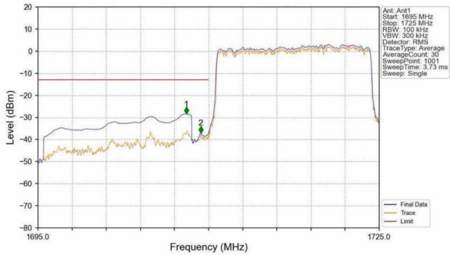
Band4 15MHz QPSK LCH 1717.5MHz RB 75 0 NTNV
