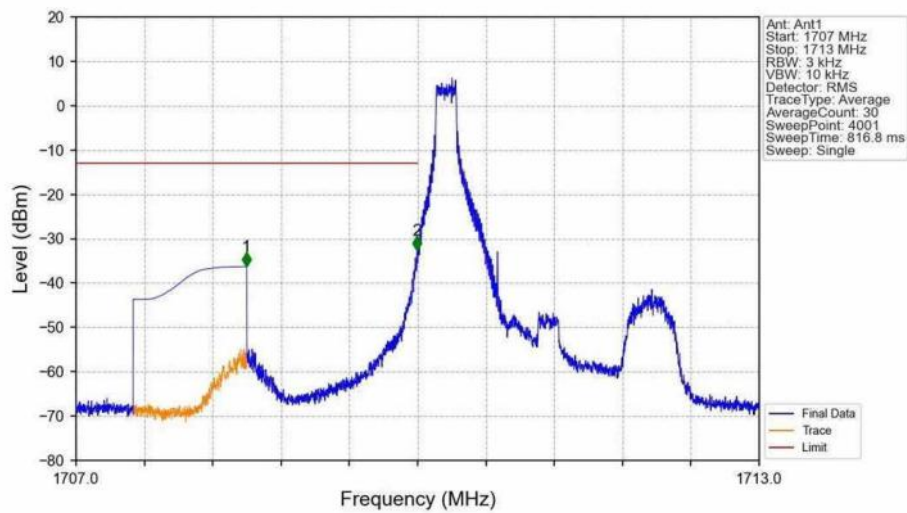
Band4 1.4MHz 16QAM LCH 1710.7MHz RB 1 0 NTNV
