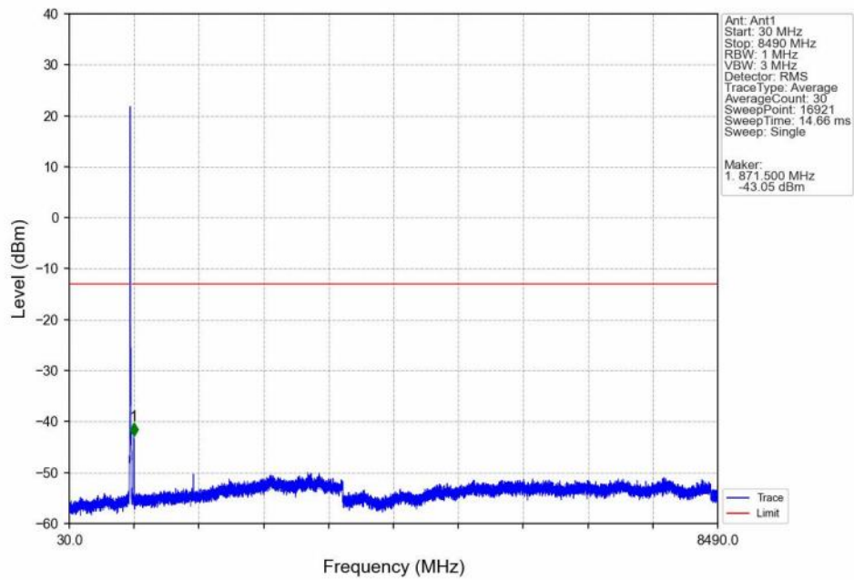
Band5 10MHz QPSK LCH 829MHz RB 50 0 NTN
