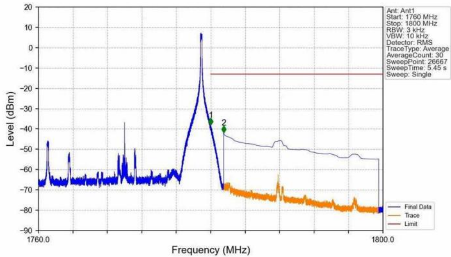
Band66_20MHz_QPSK_HCH_1770MHz_RB_1_99_NTNV
