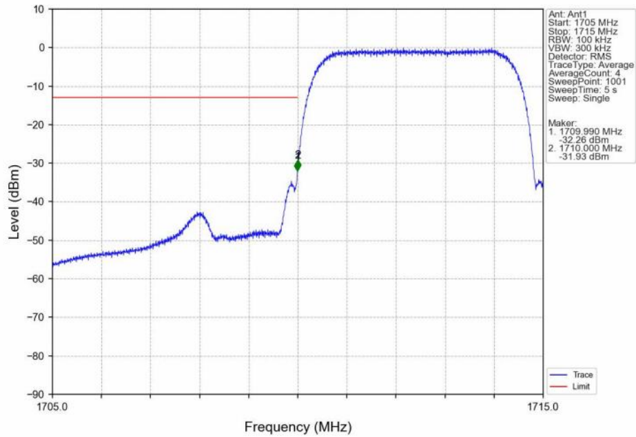
Band4_HSUPA_LCH_1712.4MHz_Subtest 1_NTNV
