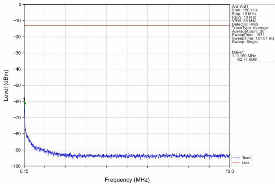
Band2_20MHz_16QAM_HCH_1900MHz_RB_1_0_NTNV
