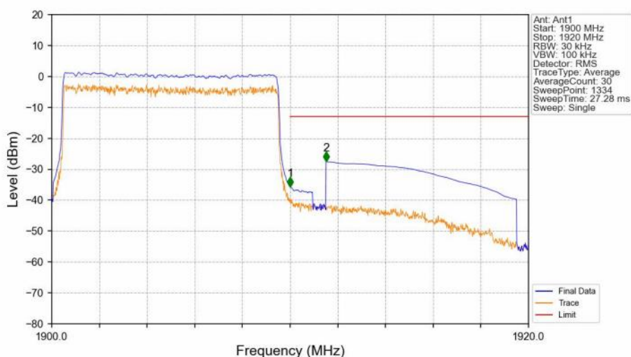
Band2_10MHz_16QAM_HCH_1905MHz_RB_50_0_NTNV
