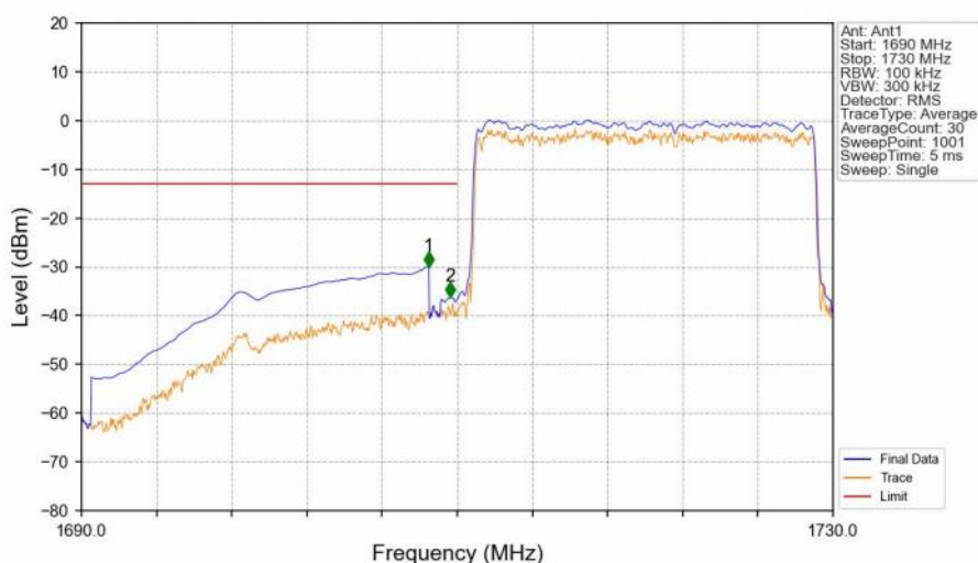
Band4_20MHz_16QAM_LCH_1720MHz_RB_100_0_NTNV
