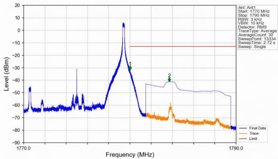
Band66_10MHz_QPSK_HCH_1775MHz_RB_1_49_NTNV
