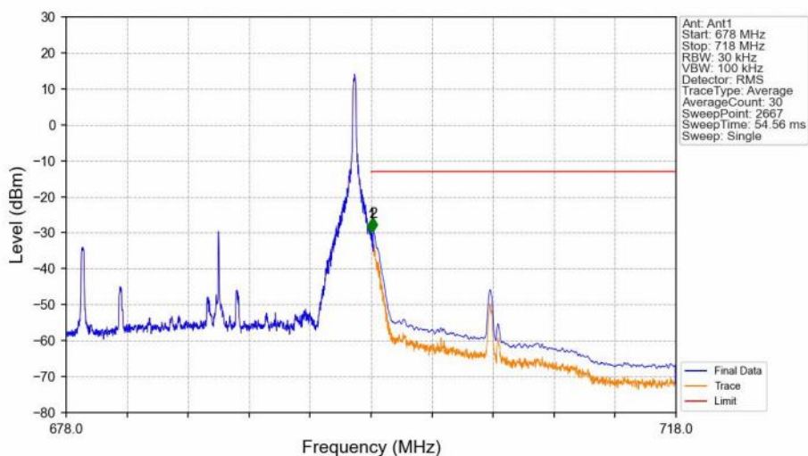
Band71_20MHz_16QAM_HCH_688MHz_RB_1_99_NTNV
