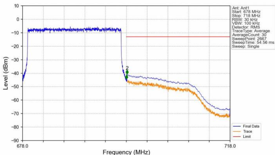
Band71_20MHz_16QAM_HCH_688MHz_RB_100_0_NTNV
