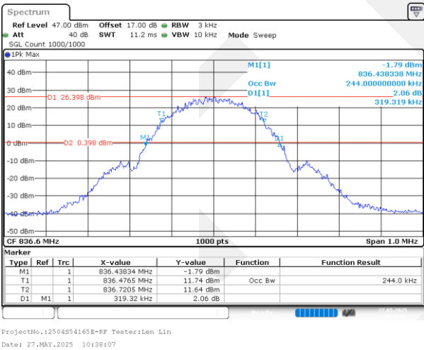
GPRS_Middle_GMSK
