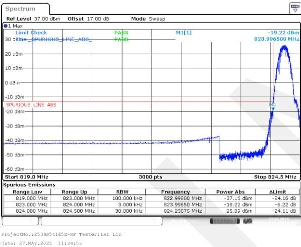
GPRS_Low_GMSK
