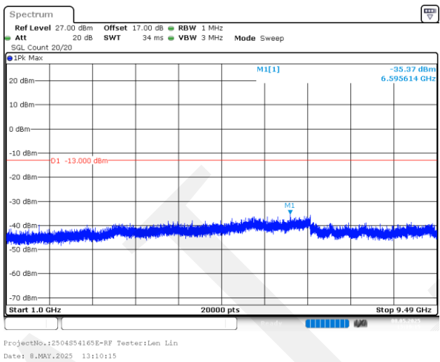
10MHz_Low_QPSK_50@0(1GHz~9.49GHz)
