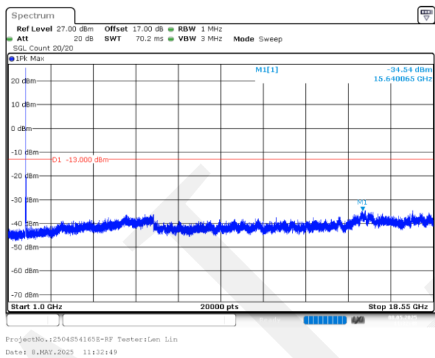
10MHz_Low_QPSK_50@0(1GHz~18.55GHz)
