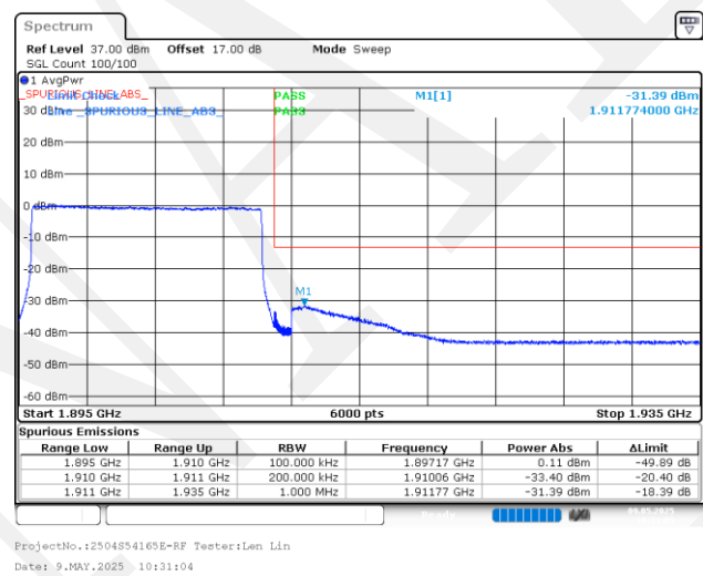
20MHz_Low_QPSK_100@0
