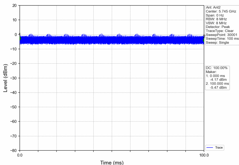
802.11a_LCH_5745MHz_Ant2_NTNV
