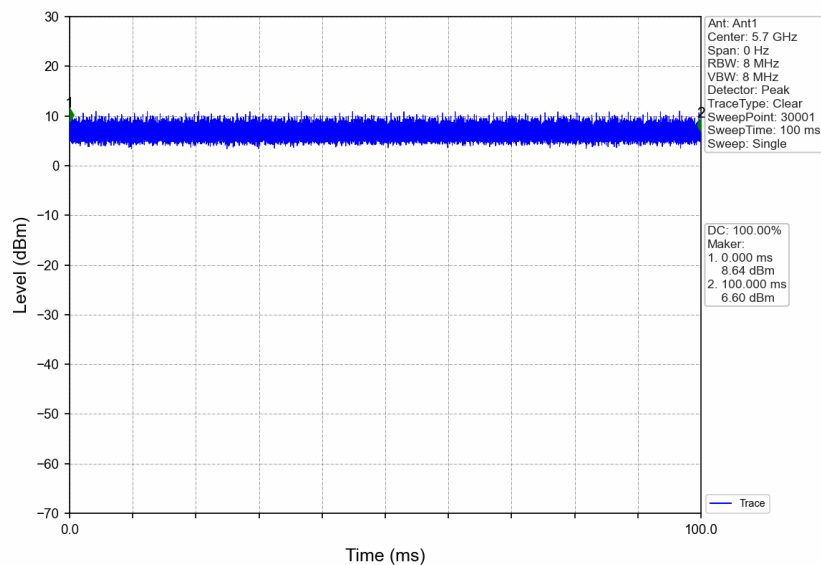
802.11n(HT20)_HCH_5700MHz_Ant1_NTNV
