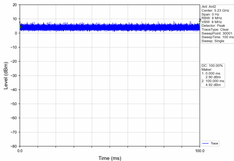
802.11n(HT40)_HCH_5230MHz_Ant2_NTNV
