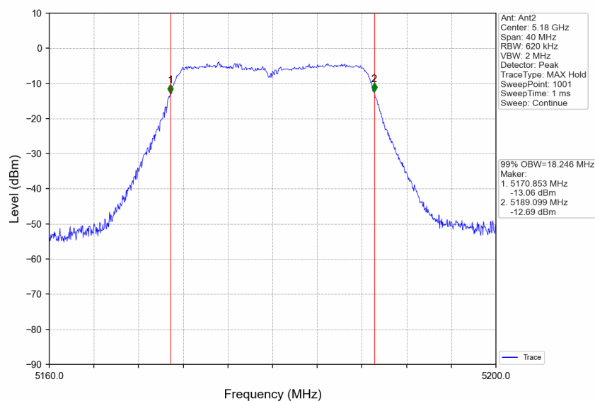
802.11n(HT20)_LCH_5180MHz_Ant2_NTNV
