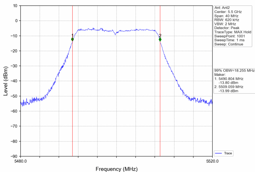
802.11n(HT20)_LCH_5500MHz_Ant2_NTNV
