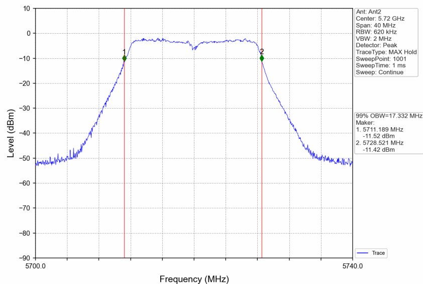
802.11a_HCH_5720MHz_Ant2_NTNV
