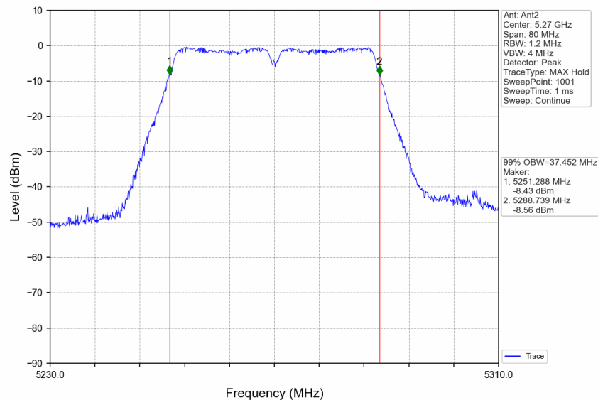
802.11ac(VHT40)_LCH_5270MHz_Ant2_NTNV
