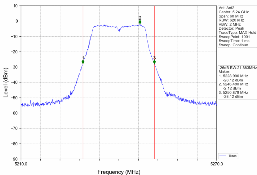
802.11a_HCH_5240MHz_Ant2_NTNV
