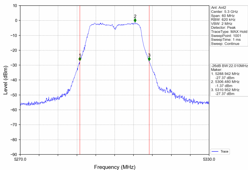
802.11a_MCH_5300MHz_Ant2_NTNV
