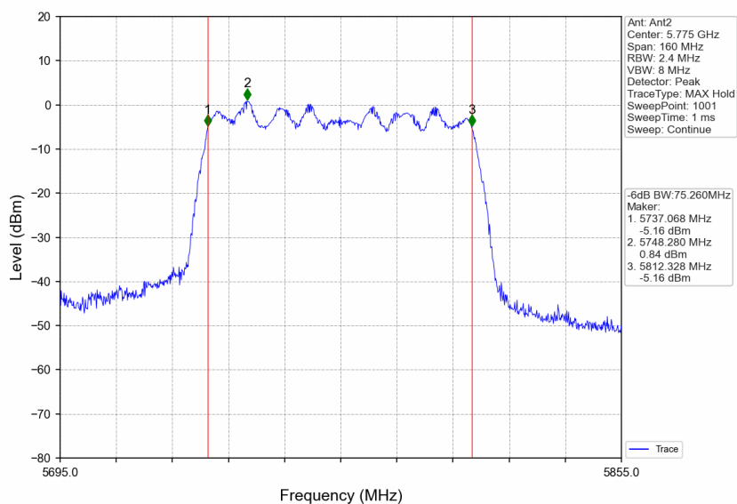
802.11ac(VHT80) MCH 5775MHz Ant2 NTNV
