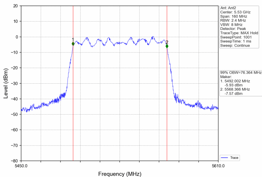
802.11ac(VHT80)_LCH_5530MHz_Ant2_NTNV
