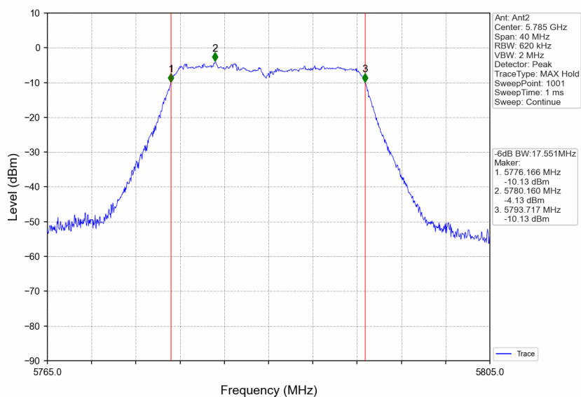
802.11n(HT20) MCH 5785MHz Ant2 NTV
