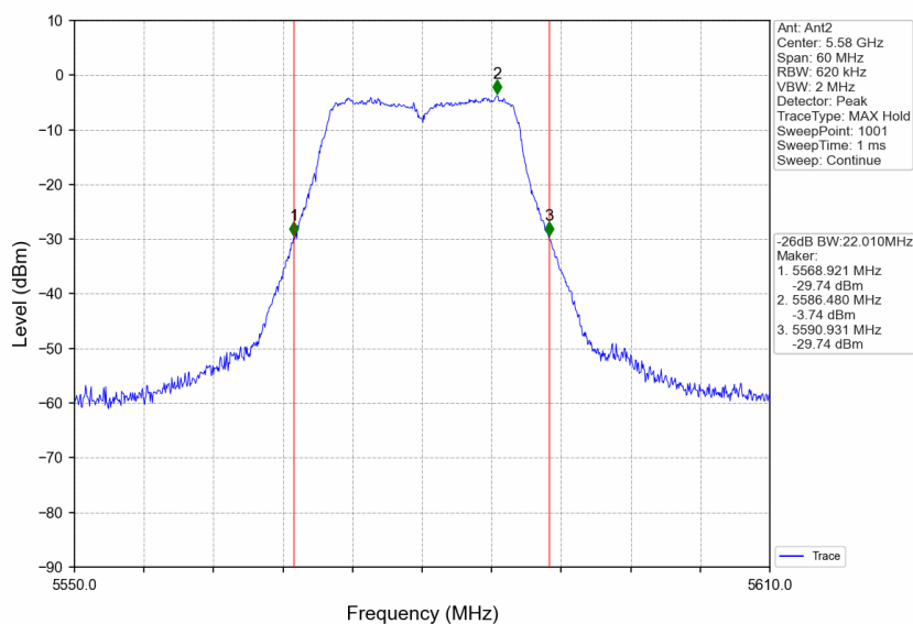
802.11a_MCH_5580MHz_Ant2_NTNV
