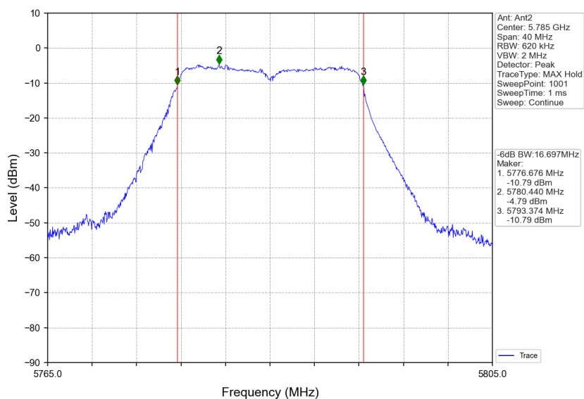
802.11a_MCH_5785MHz_Ant2_NTNV
