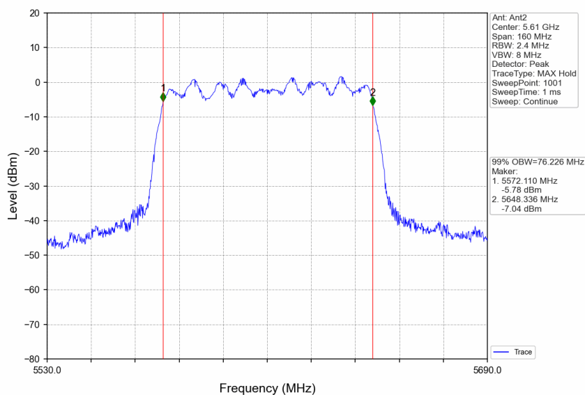
802.11ac(VHT80)_HCH_5610MHz_Ant2_NTNV
