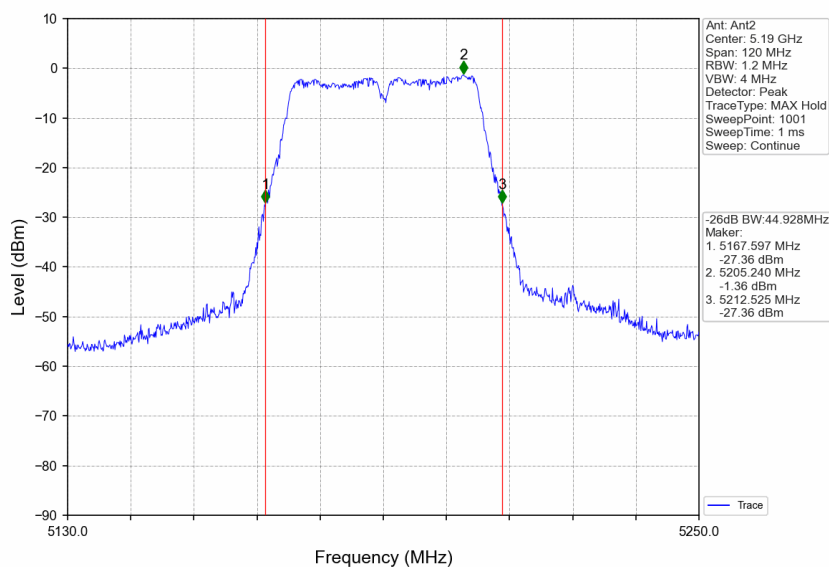
802.11n(HT40)_LCH_5190MHz_Ant2_NTNV
