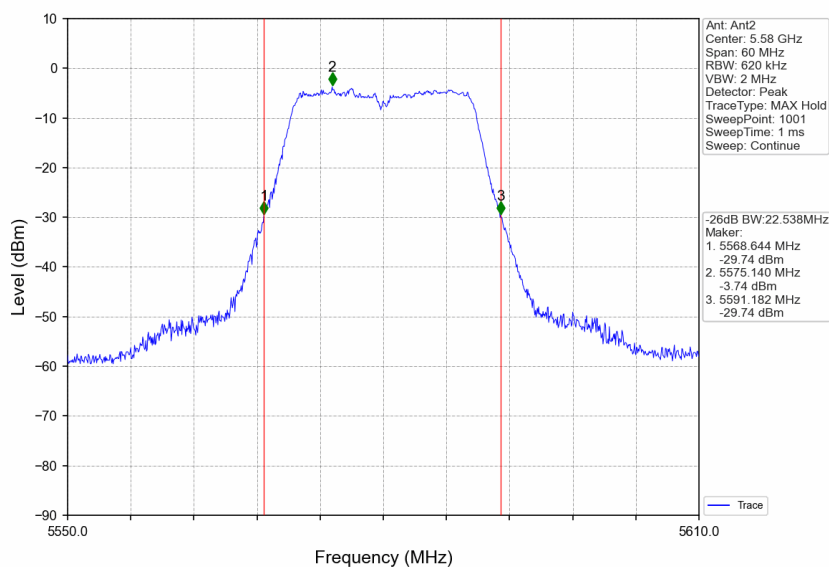
802.11n(HT20) MCH 5580MHz Ant2 NTV
