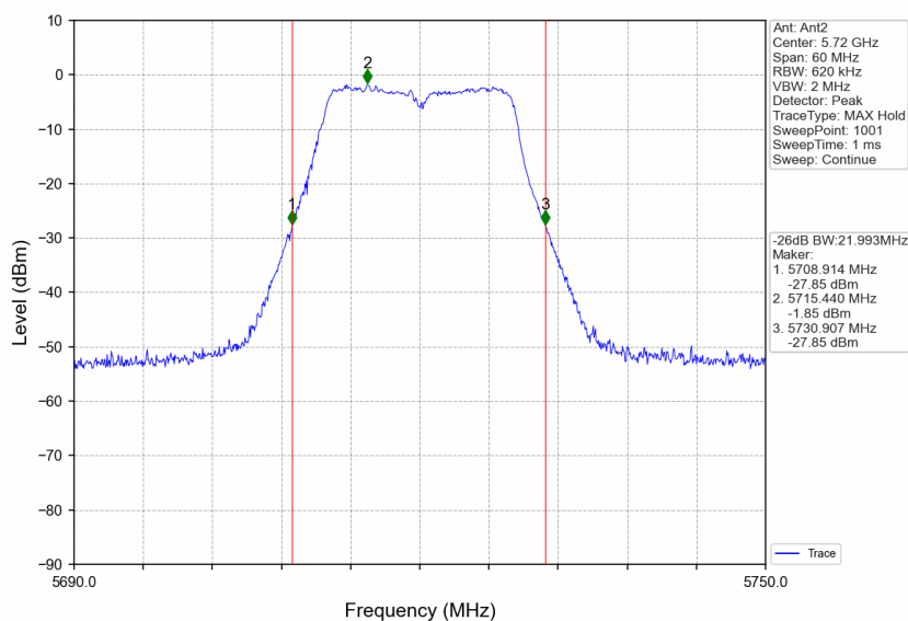
802.11a_HCH_5720MHz_Ant2_NTNV
