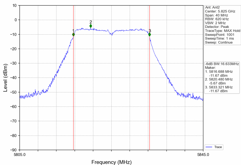
802.11a_HCH_5825MHz_Ant2_NTNV
