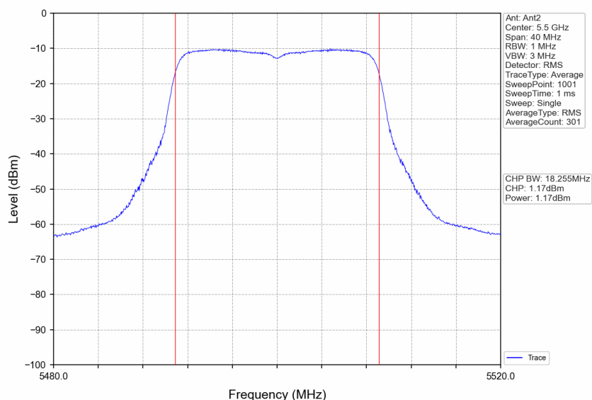
802.11n(HT20)_LCH_5500MHz_Ant2_NTNV
