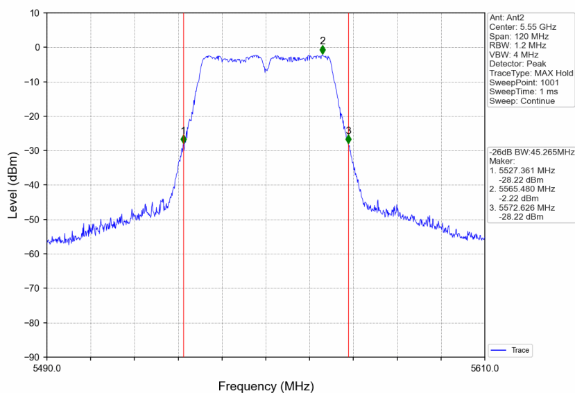
802.11n(HT40) MCH 5550MHz_Ant2_NTNV
