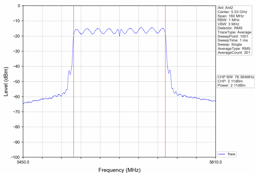
802.11ac(VHT80)_LCH_5530MHz_Ant2_NTNV
