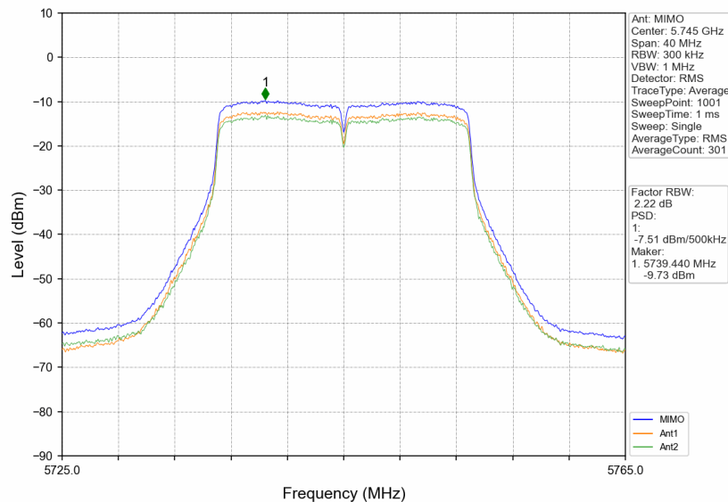
802.11ac(VHT20) LCH 5745MHz MIMO_NTNV
