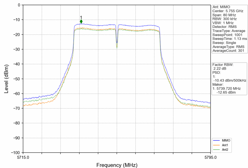
802.11n(HT40)_LCH_5755MHz_MIMO_NTNV
