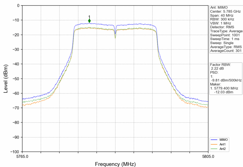
802.11n(HT20) MCH_5785MHz_MIMO_NTNV
