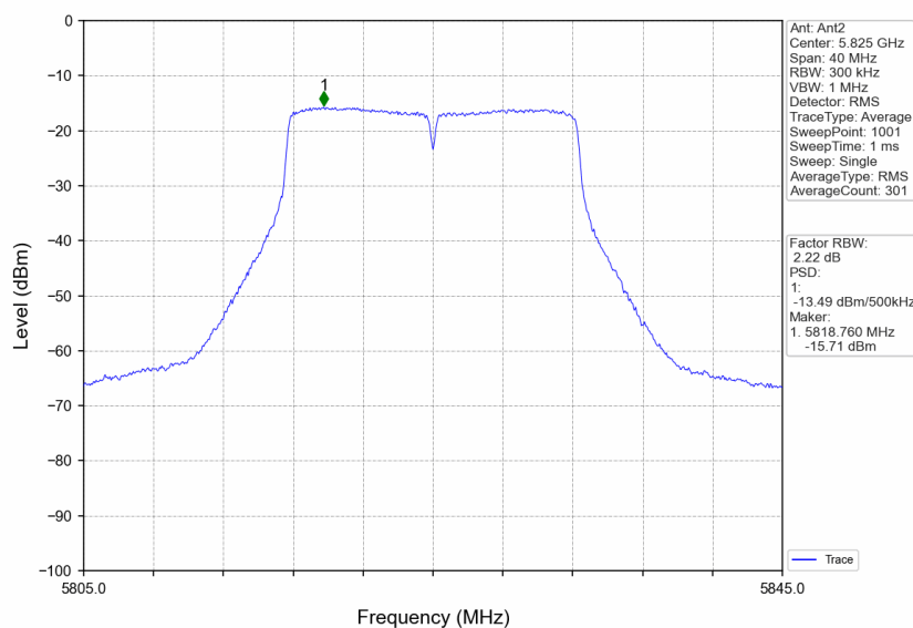
802.11a_HCH_5825MHz_Ant2_NTNV
