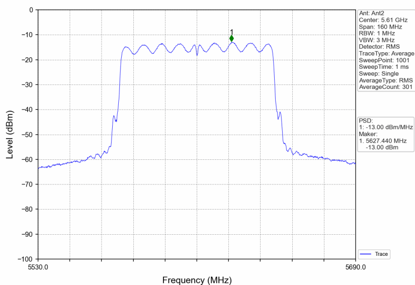
802.11ac(VHT80)_HCH_5610MHz_MIMO_NTNV
