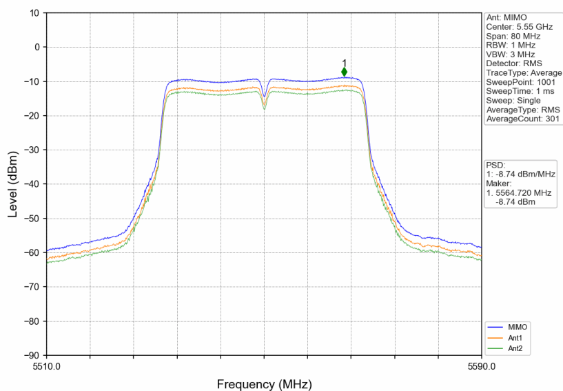
802.11ac(VHT40) MCH 5550MHz MIMO_NTNV
