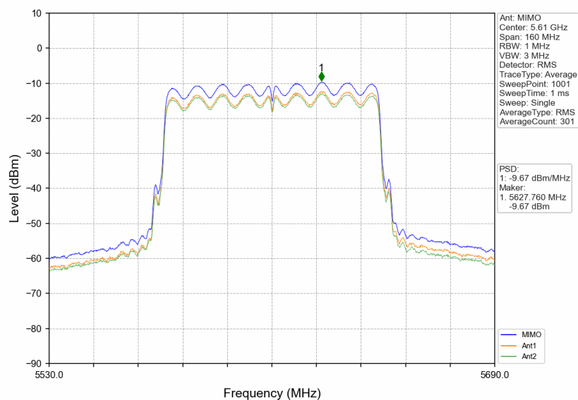
802.11ac(VHT80)_HCH_5610MHz_MIMO_NTNV
