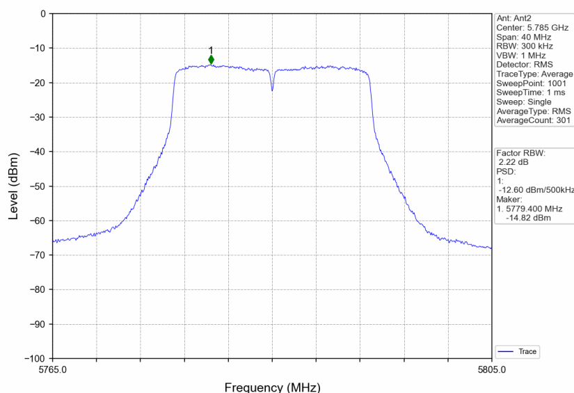
802.11n(HT20) MCH_5785MHz_MIMO_NTNV
