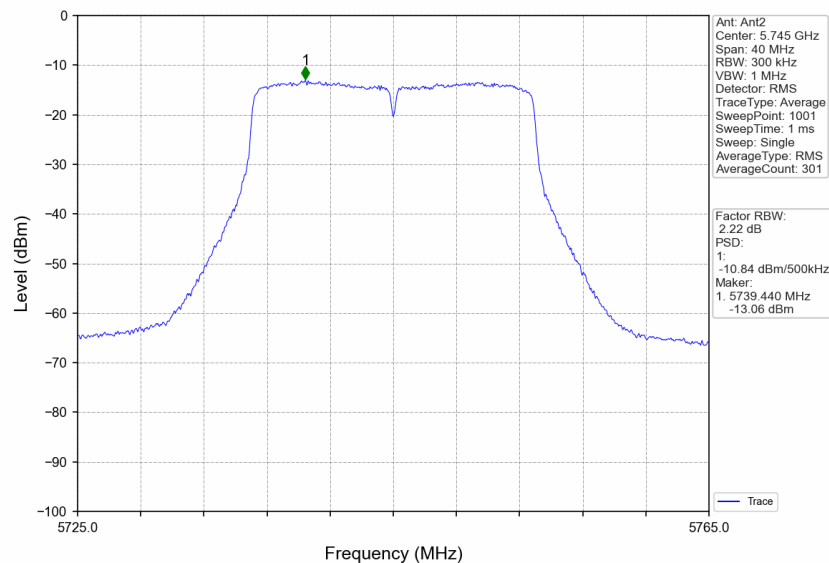
802.11ac(VHT20) LCH 5745MHz MIMO_NTNV
