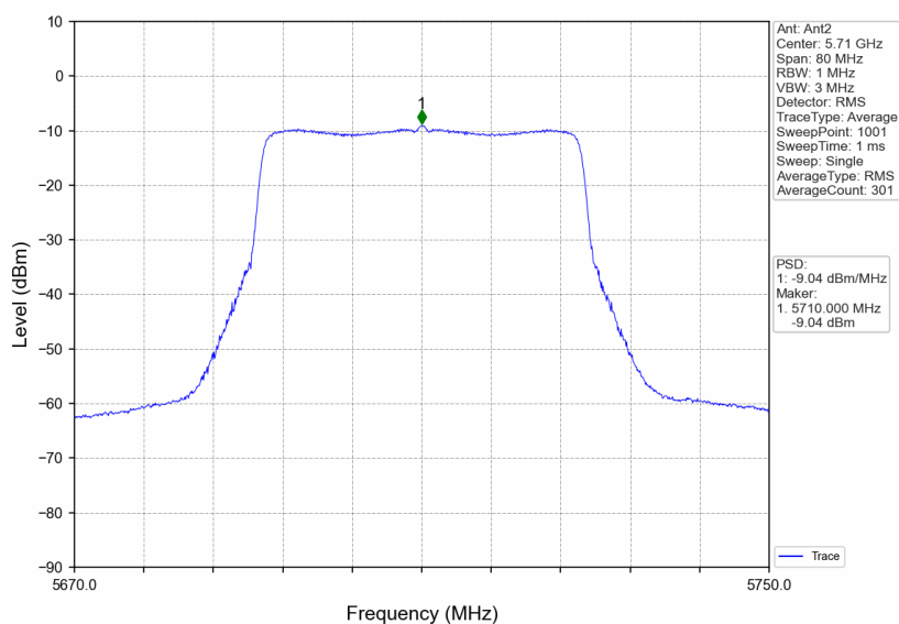
802.11ac(VHT40) HCH 5710MHz MIMO_NTNV
