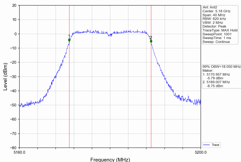
802.11n(HT20)_LCH_5180MHz_Ant2_NTNV
