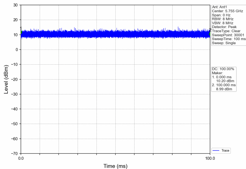
802.11n(HT40)_LCH_5755MHz_Ant1_NTNV
