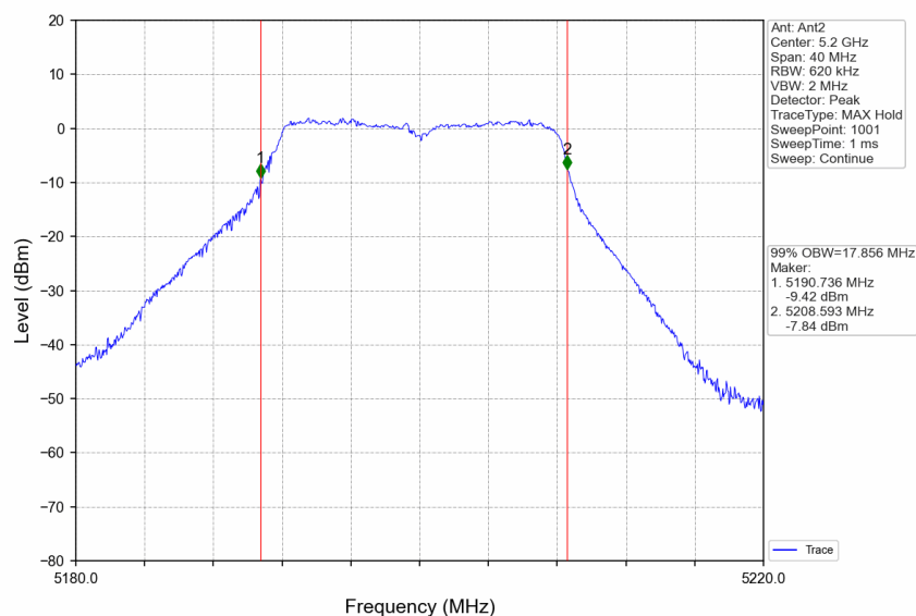
802.11a_MCH_5200MHz_Ant2_NTNV
