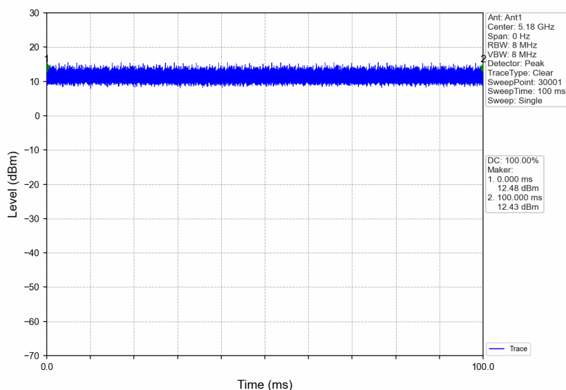
802.11n(HT20)_LCH_5180MHz_Ant1_NTNV
