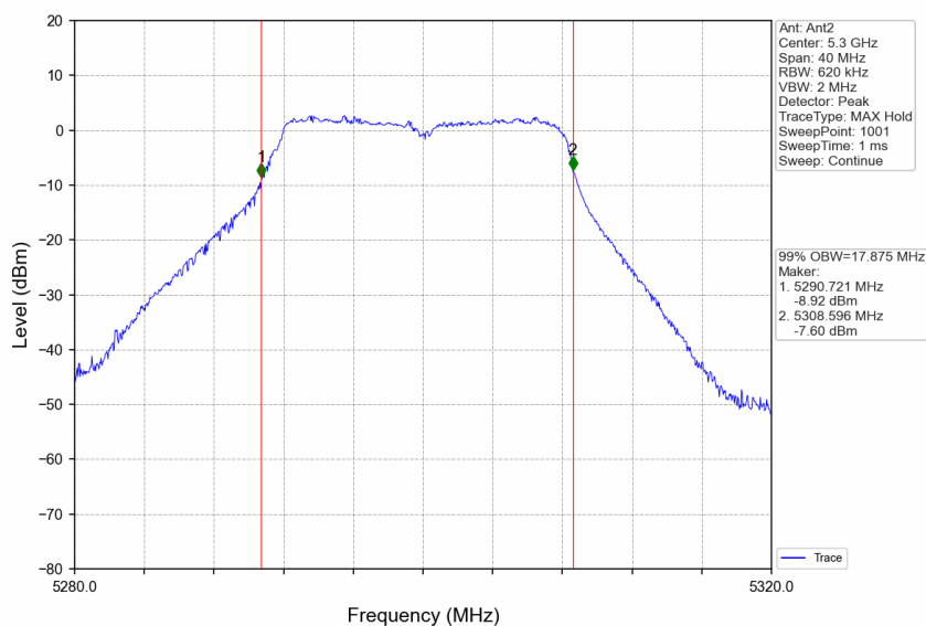
802.11a_MCH_5300MHz_Ant2_NTNV
