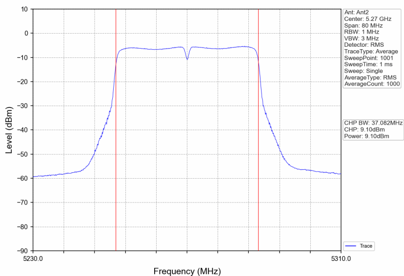
802.11n(HT40)_LCH_5270MHz_Ant2_NTNV
