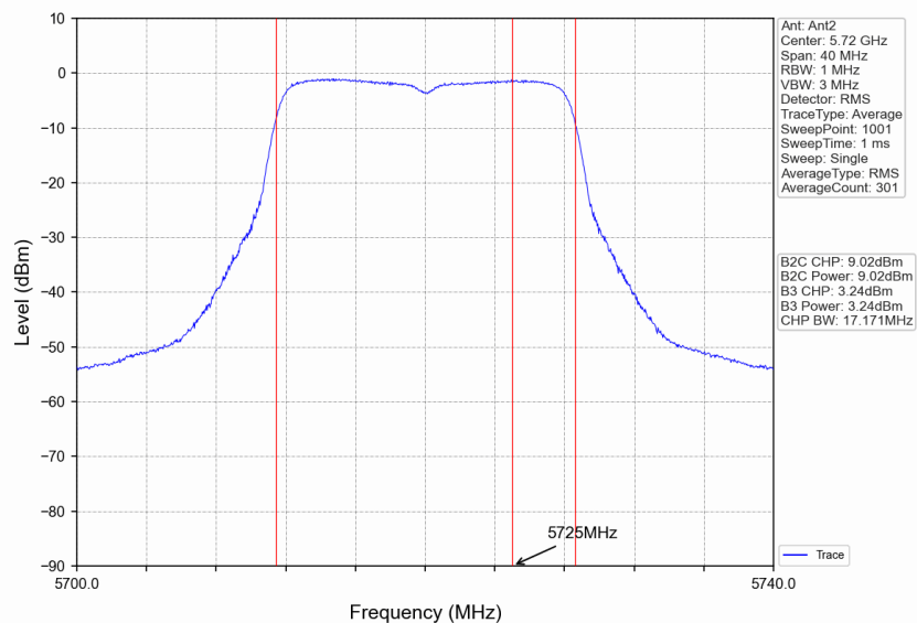
802.11a_HCH_5720MHz_Ant2_NTNV
