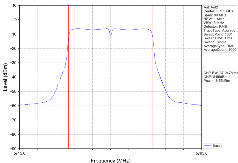
802.11n(HT40)_LCH_5755MHz_Ant2_NTNV
