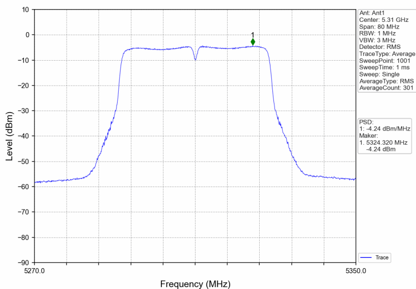
802.11n(HT40)_HCH_5310MHz_Ant1_NTNV
