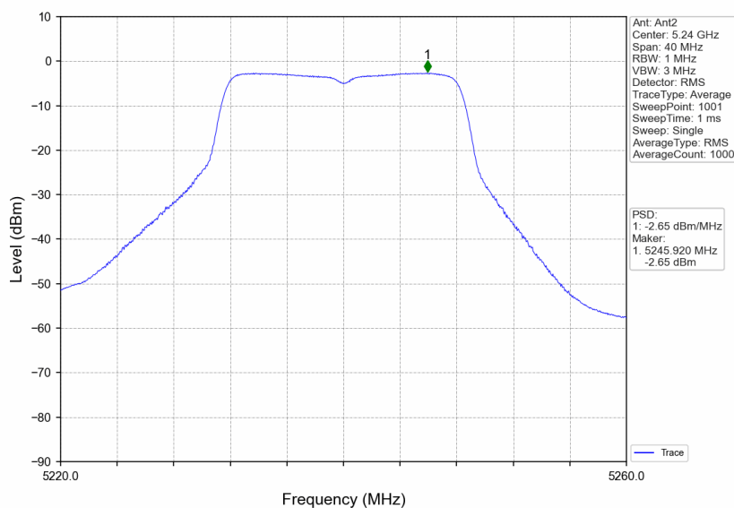
802.11a_HCH_5240MHz_Ant2_NTNV
