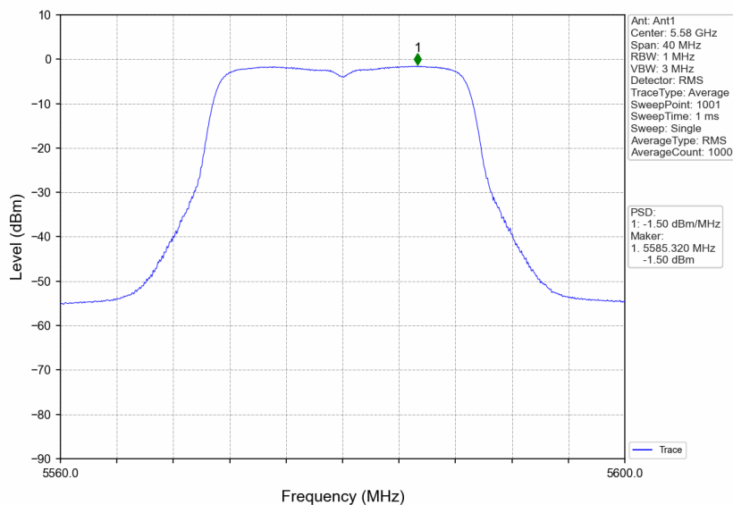
802.11n(HT20)_MCH_5580MHz_Ant1_NTNV
