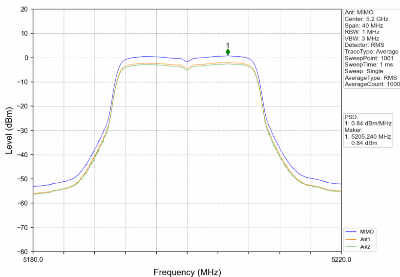
802.11n(HT20)_MCH_5200MHz_MIMO_NTNV
