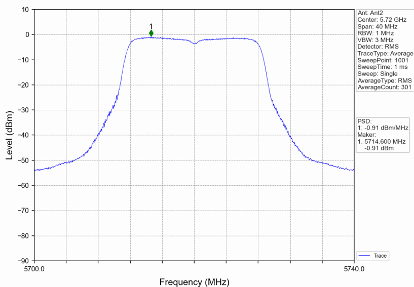
802.11a_HCH_5720MHz_Ant2_NTNV
