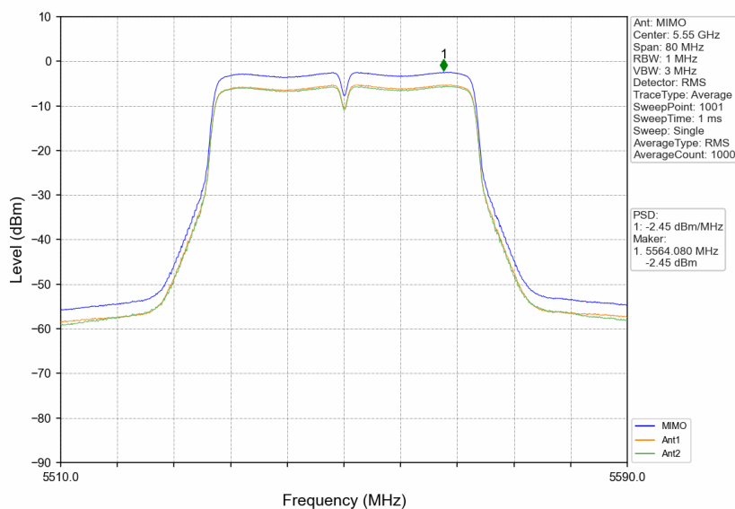
802.11n(HT40)_MCH_5550MHz_MIMO_NTNV
