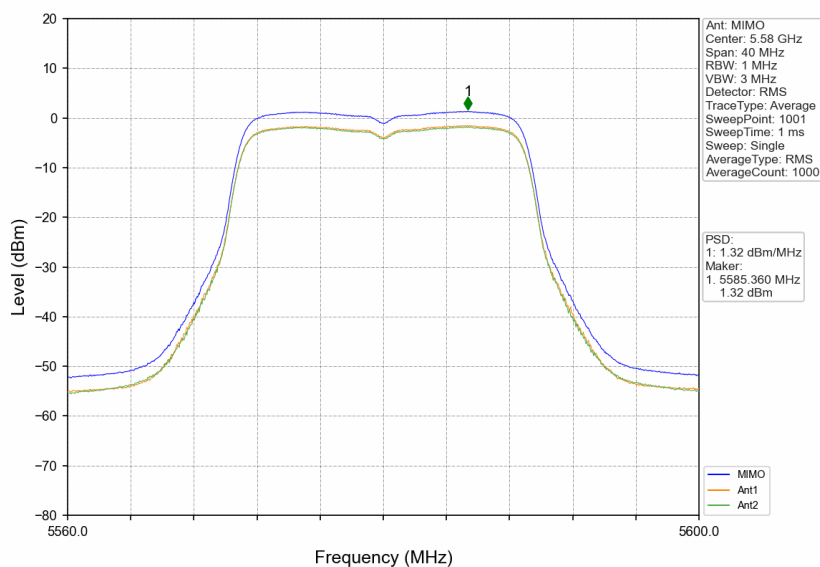
802.11n(HT20)_MCH_5580MHz_MIMO_NTNV
