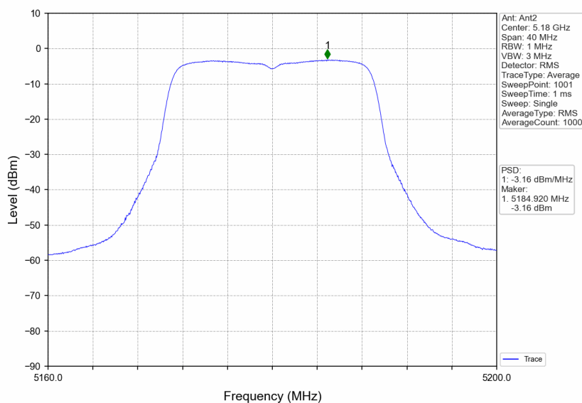
802.11n(HT20)_LCH_5180MHz_Ant2_NTNV
