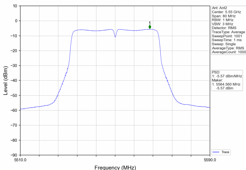
802.11n(HT40)_MCH_5550MHz_MIMO_NTNV
