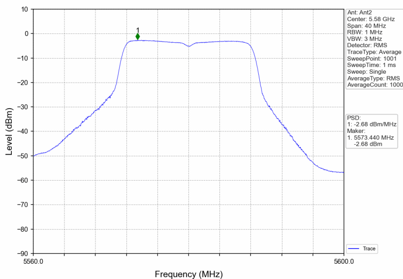
802.11a_MCH_5580MHz_Ant2_NTNV
