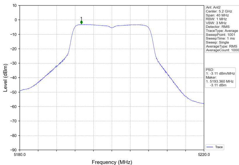
802.11a_MCH_5200MHz_Ant2_NTNV
