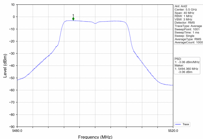
802.11a_LCH_5500MHz_Ant2_NTNV
