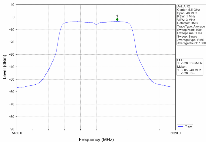
802.11ac(VHT20) LCH 5500MHz Ant2 NTNV
