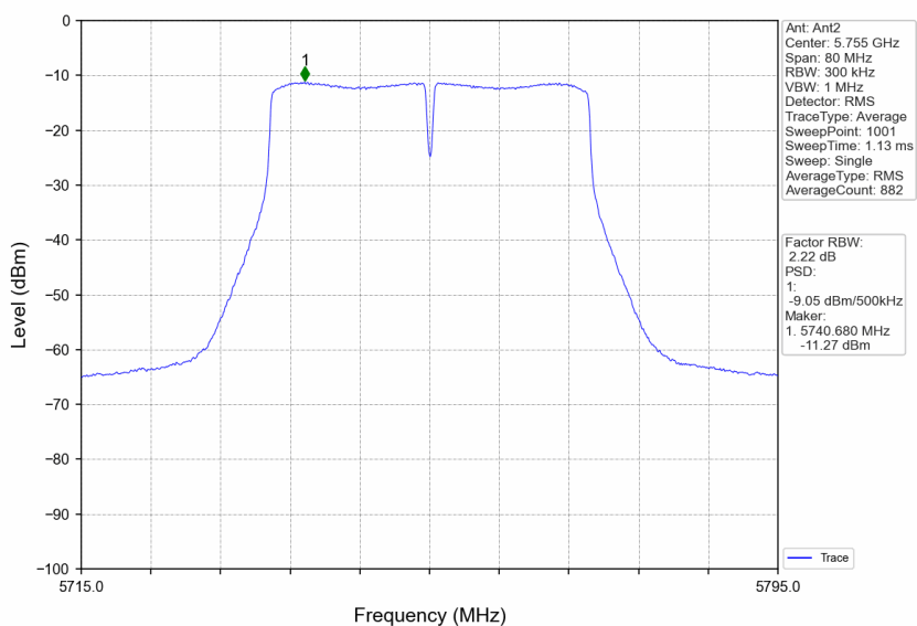
802.11ac(VHT40)_LCH_5755MHz_Ant2_NTNV
