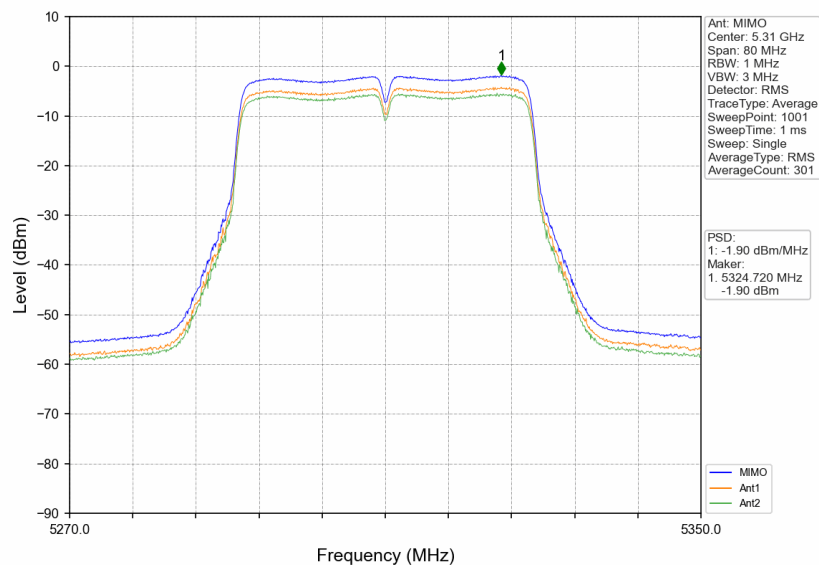
802.11ac(VHT40) HCH 5310MHz MIMO_NTNV
