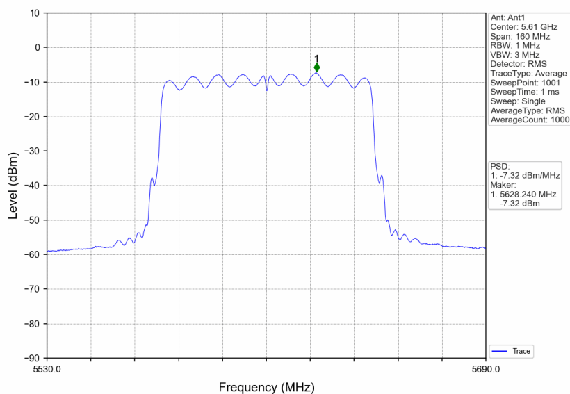
802.11ac(VHT80)_HCH_5610MHz_Ant1_NTNV
