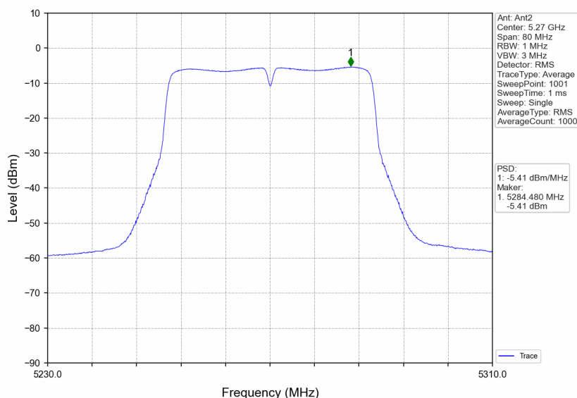
802.11ac(VHT40)_LCH_5270MHz_Ant2_NTNV
