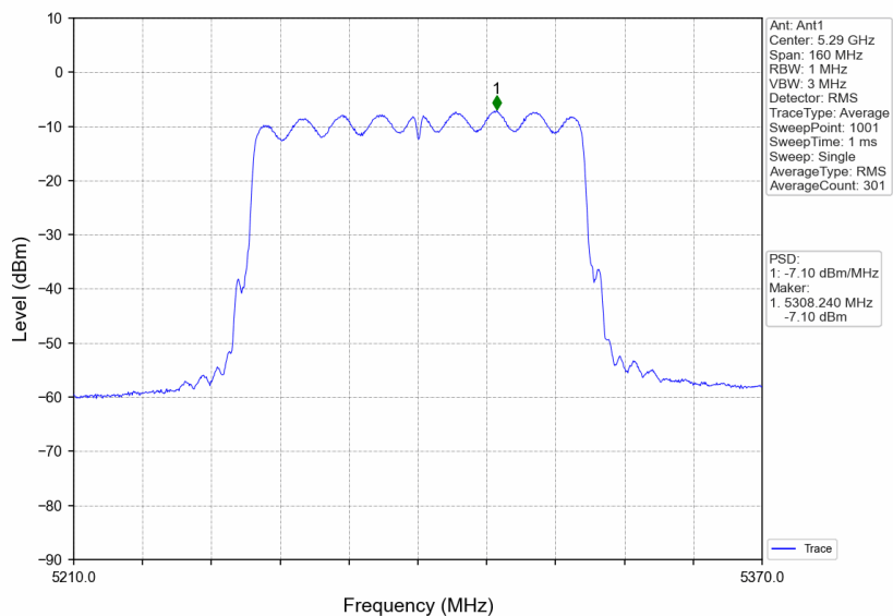
802.11ac(VHT80) MCH_5290MHz_Ant1_NTNV
