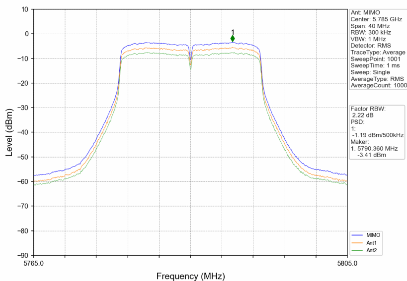
802.11n(HT20)_MCH_5785MHz_MIMO_NTNV
