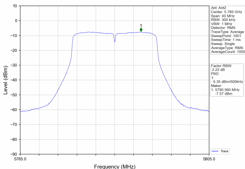
802.11n(HT20)_MCH_5785MHz_MIMO_NTNV
