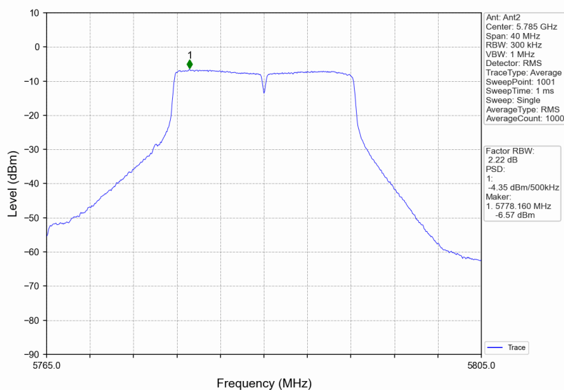
802.11a_MCH_5785MHz_Ant2_NTNV
