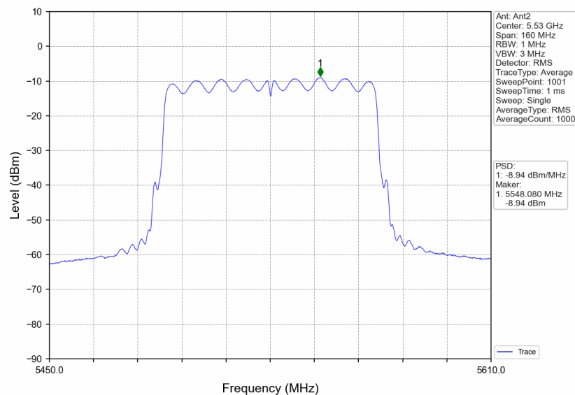
802.11ac(VHT80)_LCH_5530MHz_Ant2_NTNV
