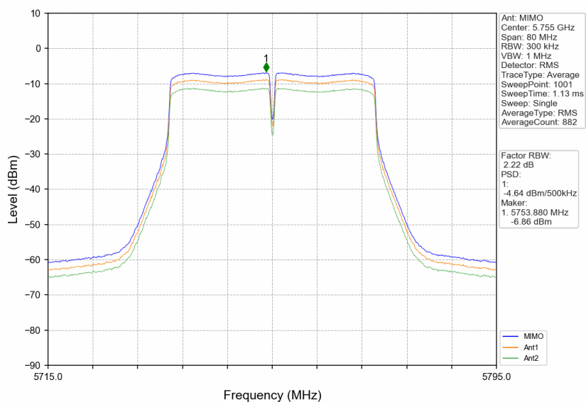
802.11n(HT40)_LCH_5755MHz_MIMO_NTNV
