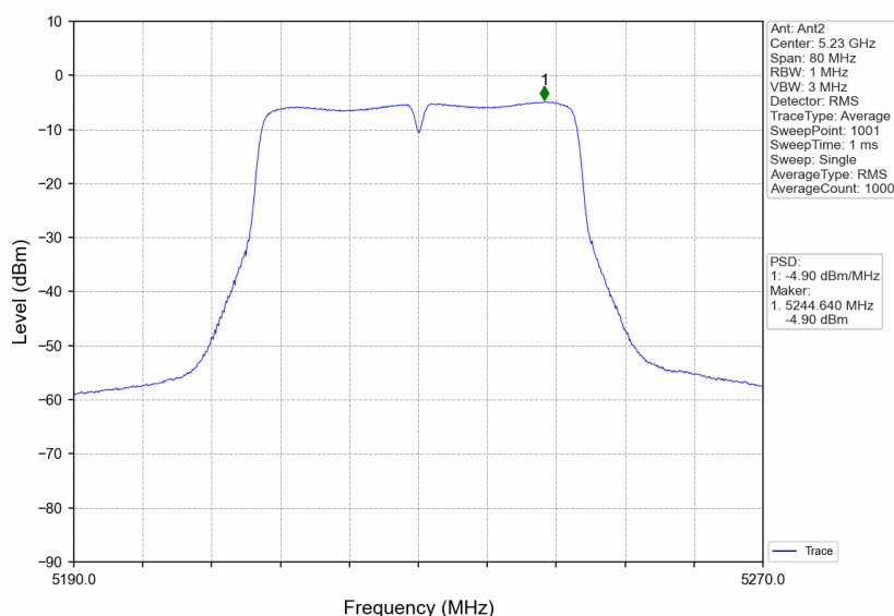
802.11ac(VHT40) HCH 5230MHz MIMO_NTNV
