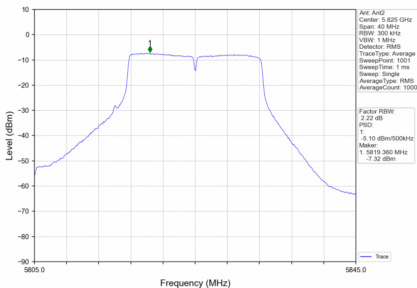
802.11a_HCH_5825MHz_Ant2_NTNV
