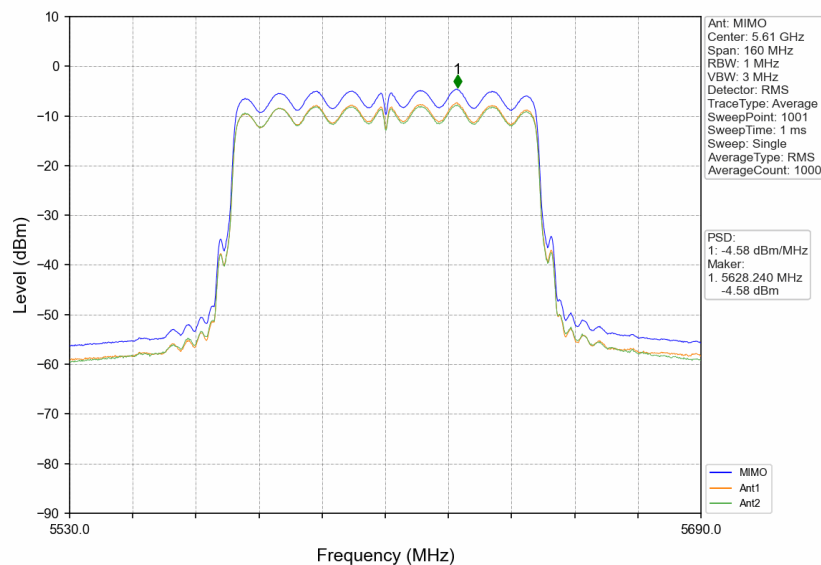
802.11ac(VHT80)_HCH_5610MHz_MIMO_NTNV
