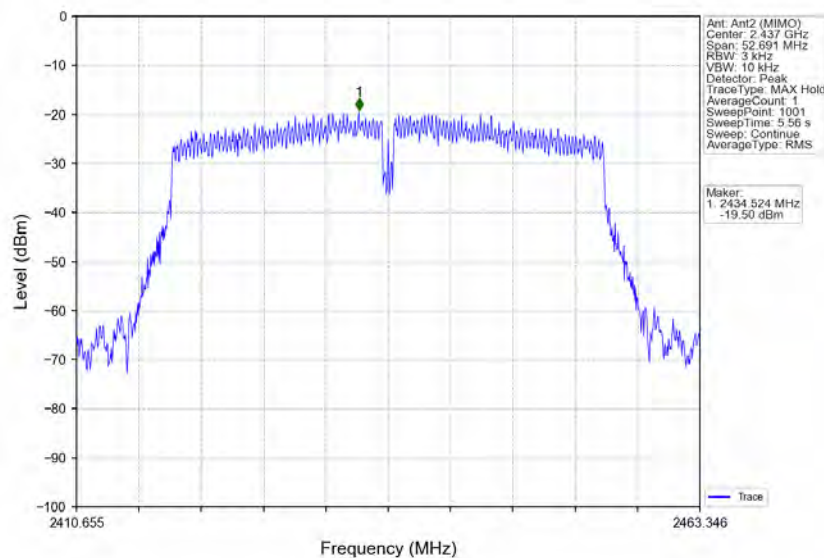
802.11n(HT40)_MCH_2437MHz_Ant2 (MIMO)_NTNV
