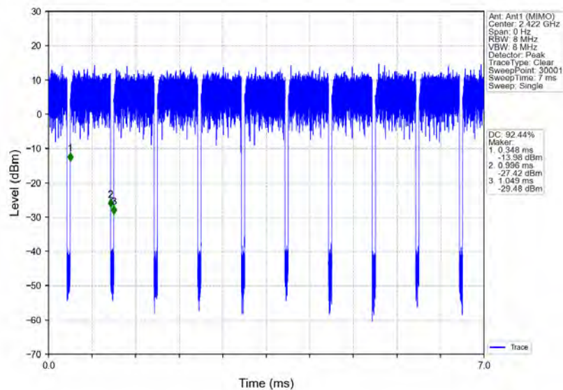
802.11n(HT40)_LCH_2422MHz_Ant1 (MIMO)_NTNV
