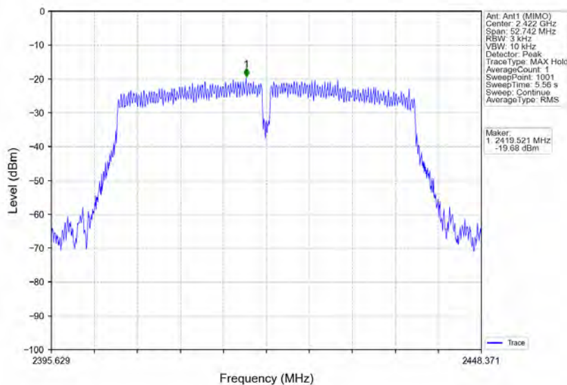
802.11n(HT40)_LCH_2422MHz_Ant1 (MIMO)_NTNV
