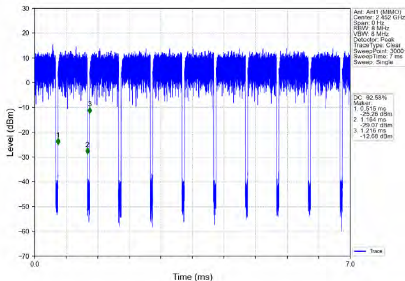
802.11n(HT40)_HCH_2452MHz_Ant1 (MIMO)_NTNV
