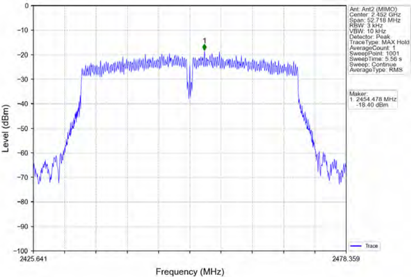
802.11n(HT40)_HCH_2452MHz_MIMO_NTNV
