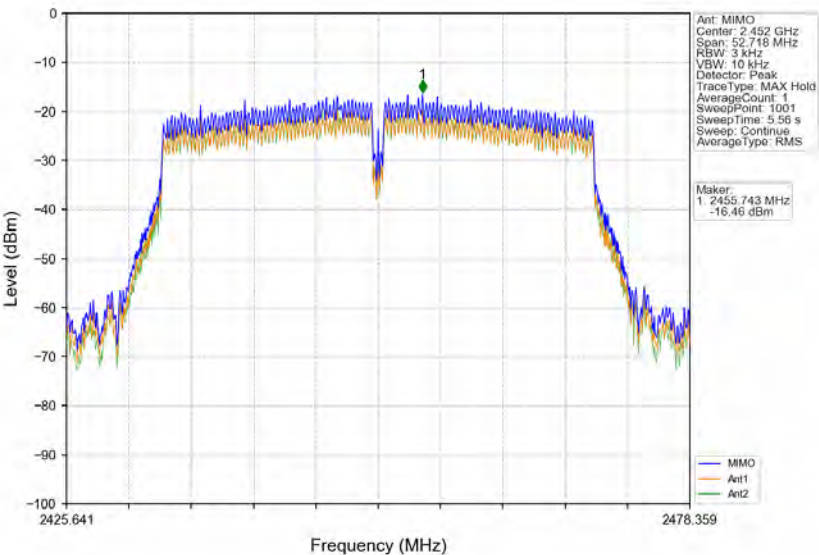
802.11n(HT40)_HCH_2452MHz_MIMO_NTNV
