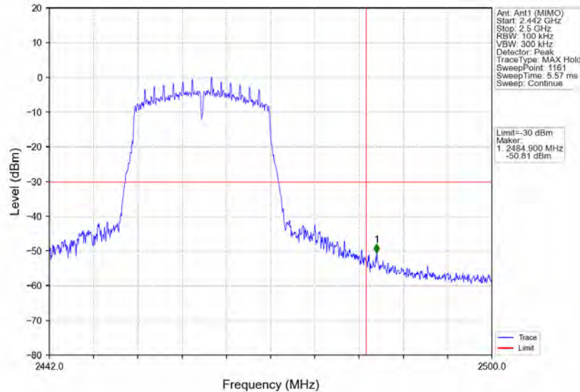
802.11n(HT20)_HCH_2462MHz_Ant1 (MIMO)_NTNV
