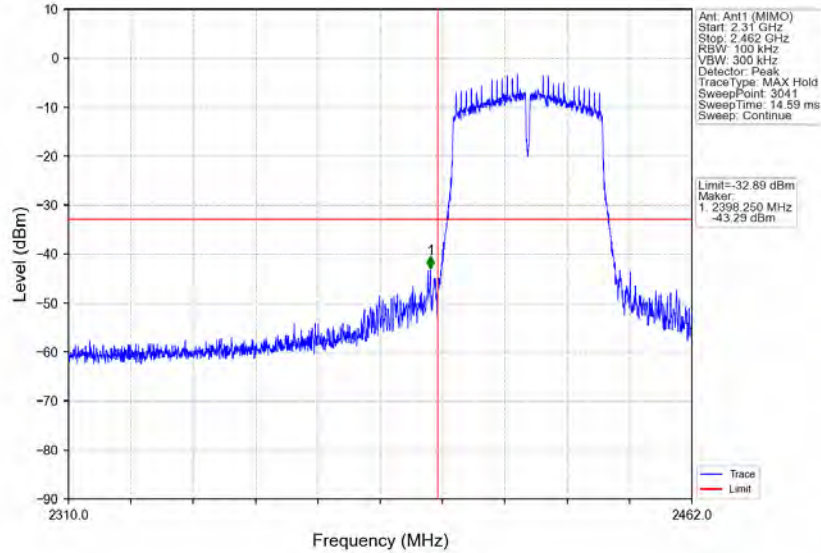
802.11n(HT40)_LCH_2422MHz_Ant1 (MIMO)_NTNV
