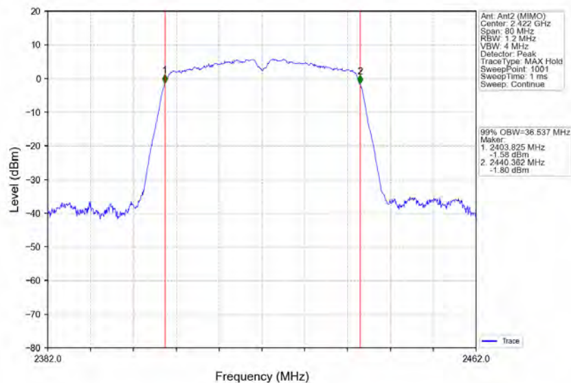
802.11n(HT40)_LCH_2422MHz_Ant2 (MIMO)_NTNV
