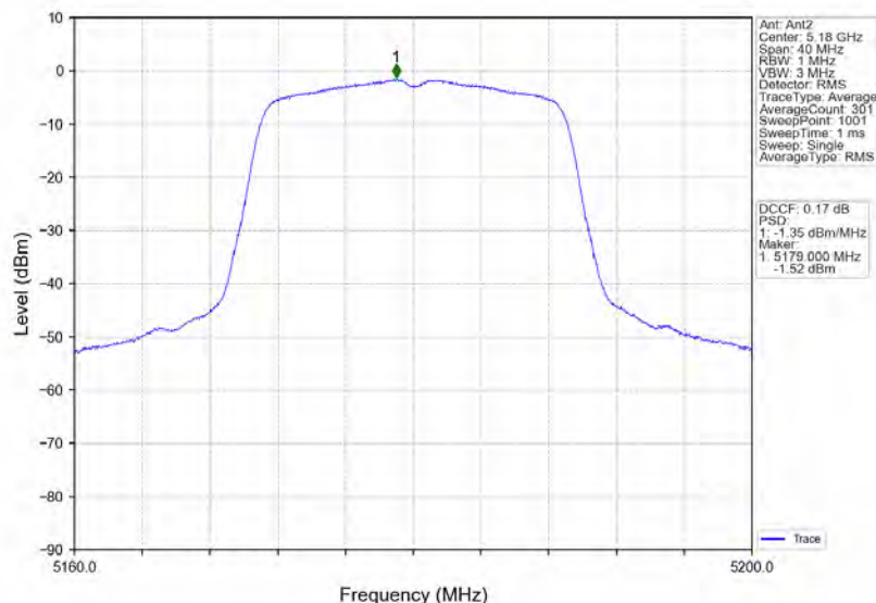
802.11n(HT20)_LCH_5180MHz_MIMO_NTNV
