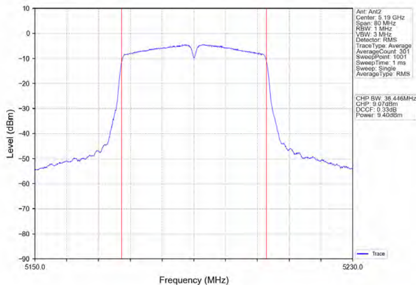
802.11n(HT40)_LCH_5190MHz_Ant2_NTNV
