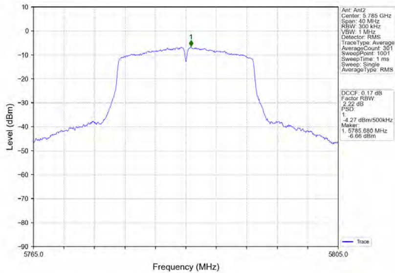
802.11n(HT20)_MCH_5785MHz_MIMO_NTNV
