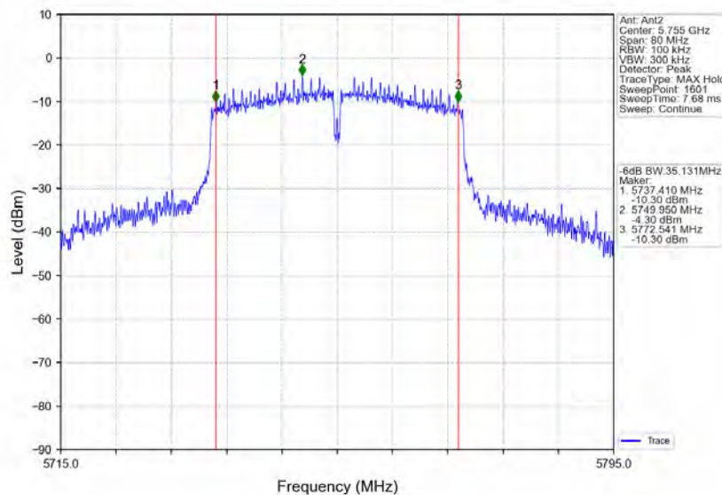
802.11n(HT40)_LCH_5755MHz_Ant2_NTNV
