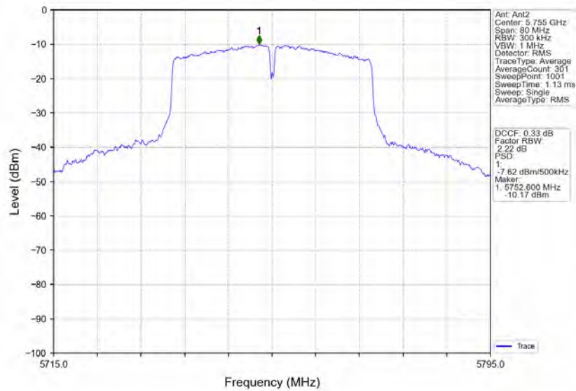
802.11n(HT40)_LCH_5755MHz_MIMO_NTNV
