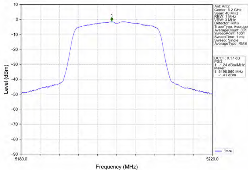
802.11n(HT20)_MCH_5200MHz_MIMO_NTNV
