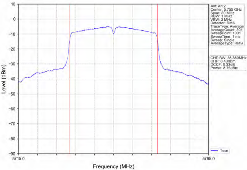
802.11n(HT40)_LCH_5755MHz_Ant2_NTNV
