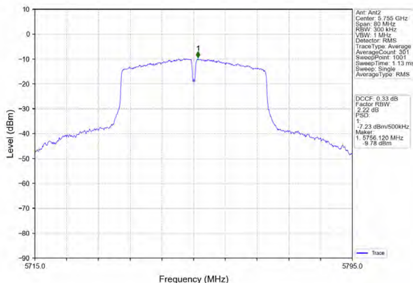
802.11ac(VHT40)_LCH_5755MHz_MIMO_NTNV
