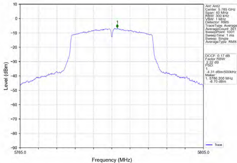
802.11n(HT20)_MCH_5785MHz_MIMO_NTNV
