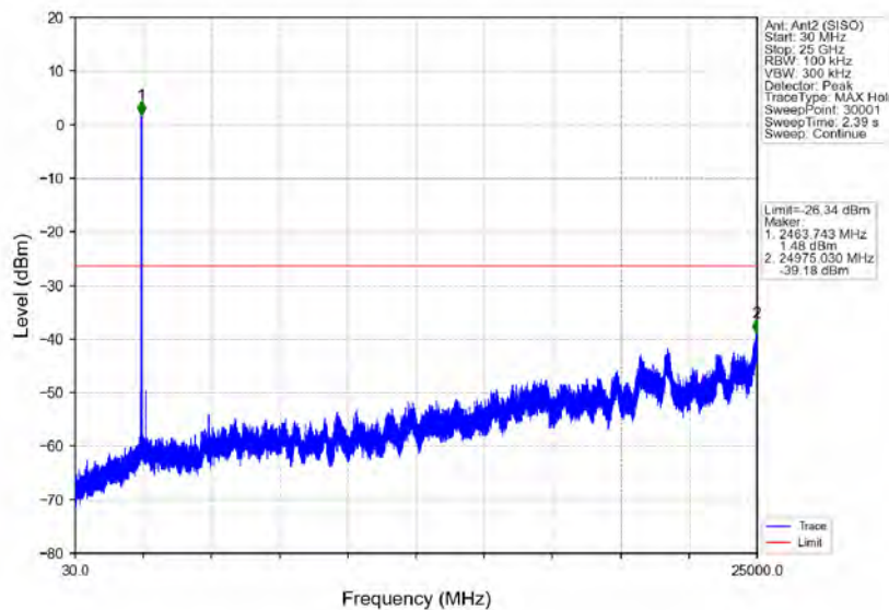
802.11b_HCH_2462MHz_Ant2 (SISO)_NTNV
