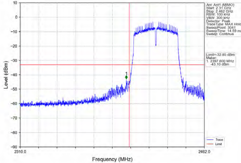
802.11n(HT40)_LCH_2422MHz_Ant1 (MIMO)_NTNV
