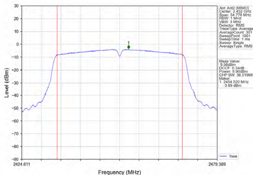
802.11n(HT40)_HCH_2452MHz_Ant2 (MIMO)_NTNV
