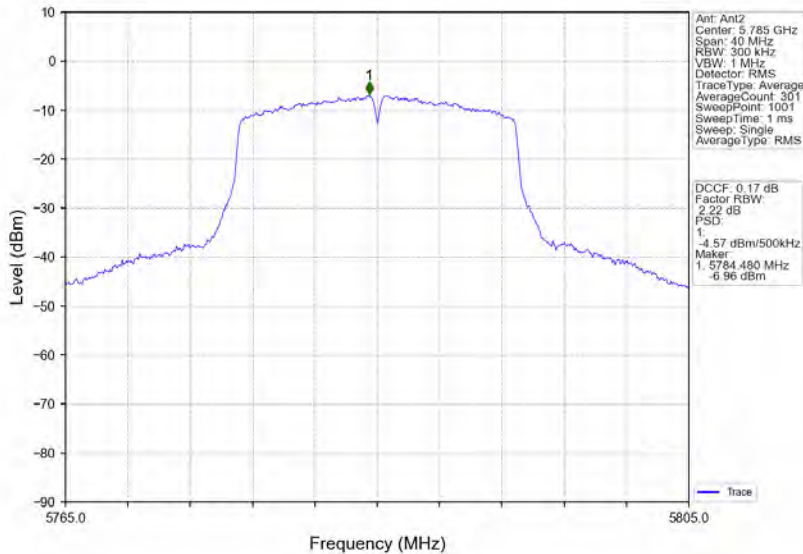
802.11n(HT20)_MCH_5785MHz_MIMO_NTNV
