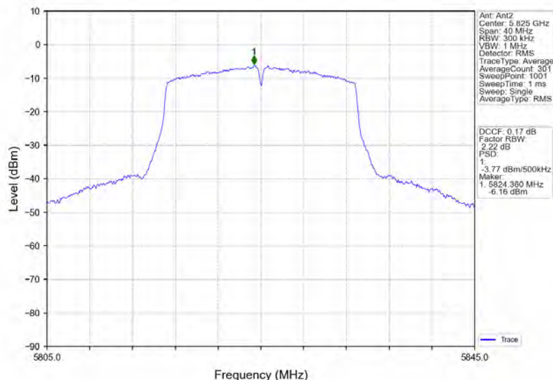
802.11n(HT20)_HCH_5825MHz_MIMO_NTNV
