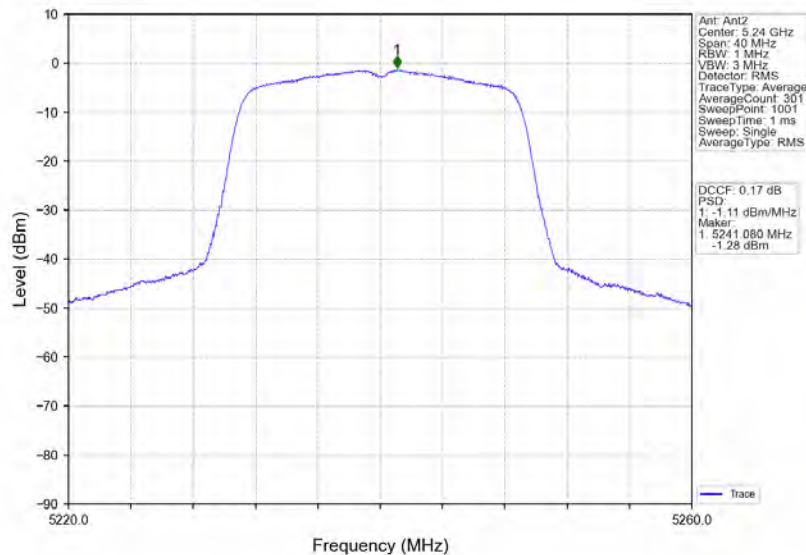
802.11n(HT20)_HCH_5240MHz_MIMO_NTNV
