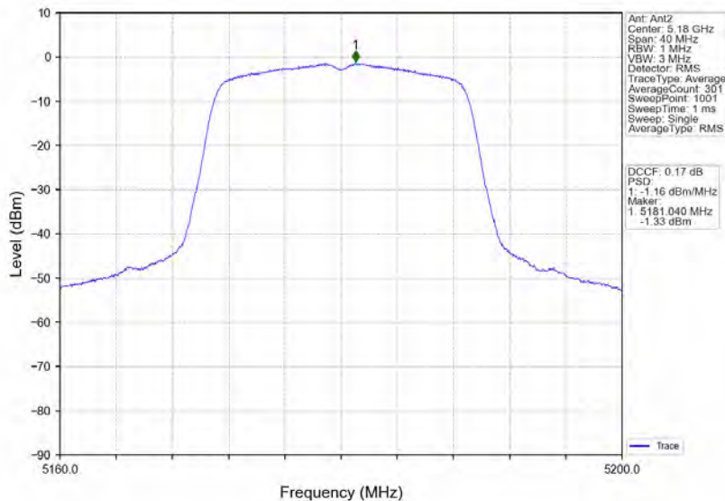
802.11n(HT20)_LCH_5180MHz_MIMO_NTNV
