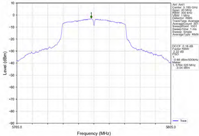
802.11a_MCH_5785MHz_Ant4_NTNV
