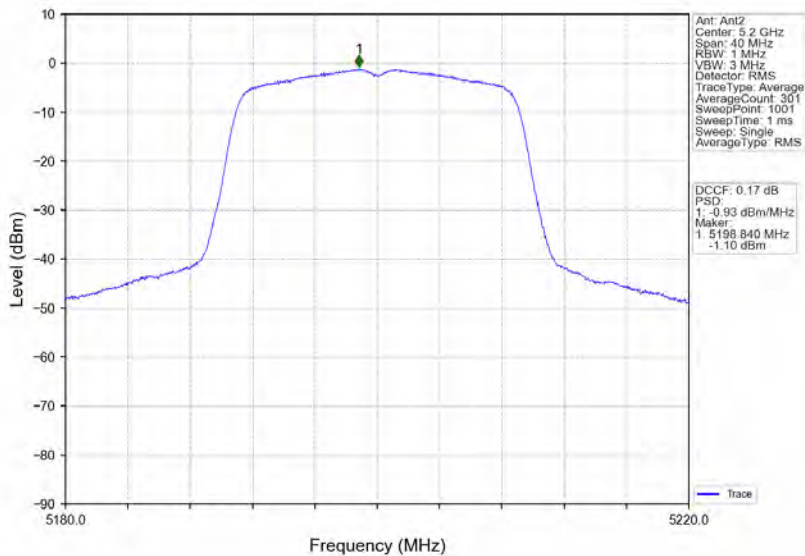
802.11n(HT20)_MCH_5200MHz_MIMO_NTNV
