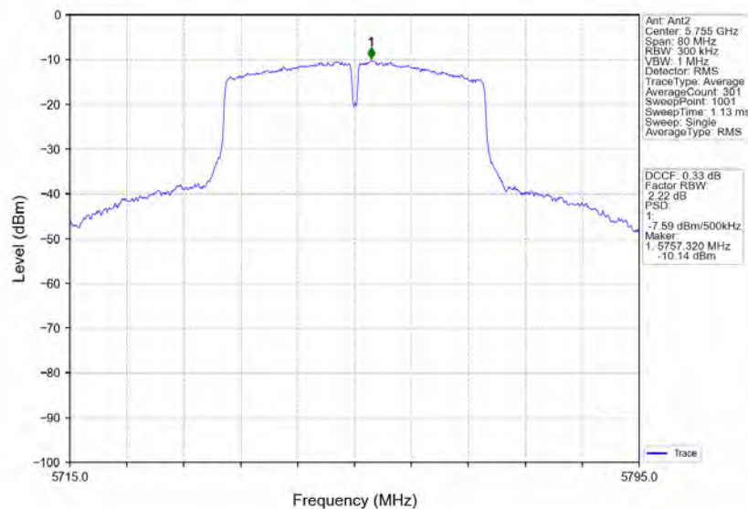
802.11ac(VHT40)_LCH_5755MHz_MIMO_NTNV
