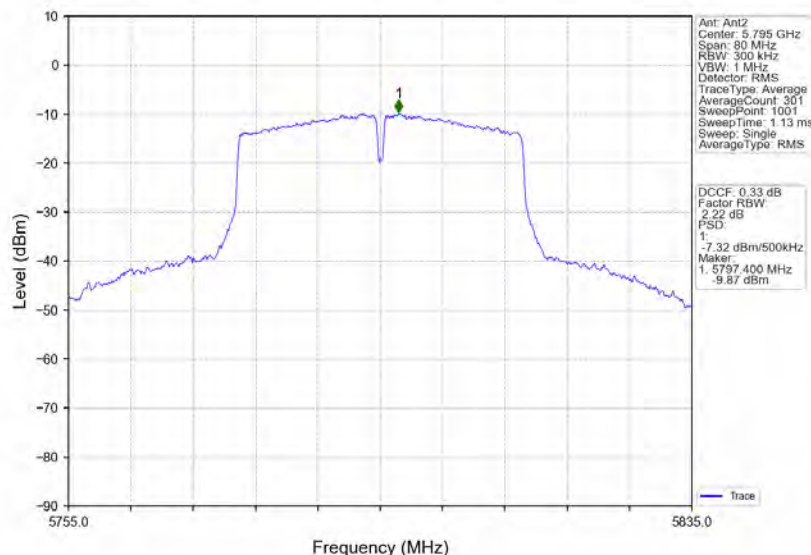
802.11n(HT40)_HCH_5795MHz_MIMO_NTNV
