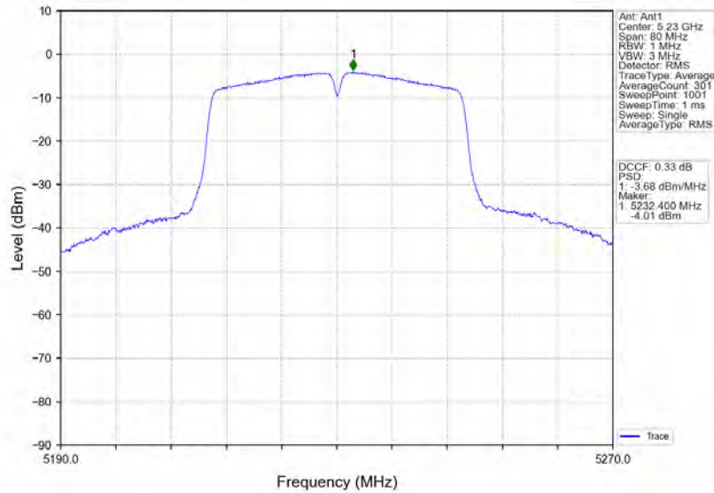
802.11n(HT40)_HCH_5230MHz_Ant4_NTNV
