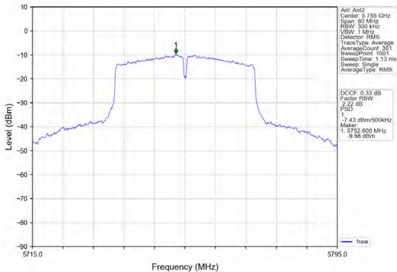
802.11n(HT40)_LCH_5755MHz_MIMO_NTNV
