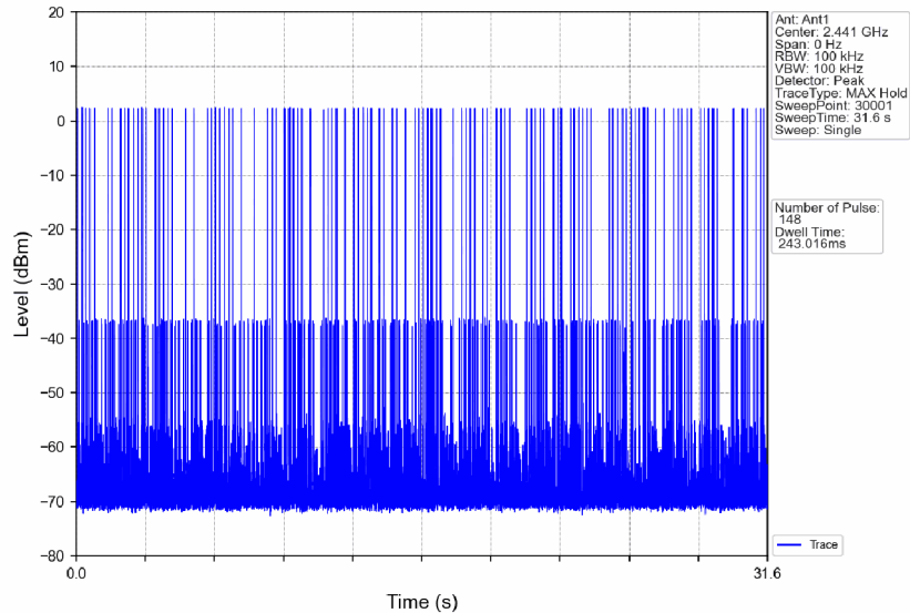
Pi/4DQPSK_2DH5_HOPP_Ant1_NTNV
