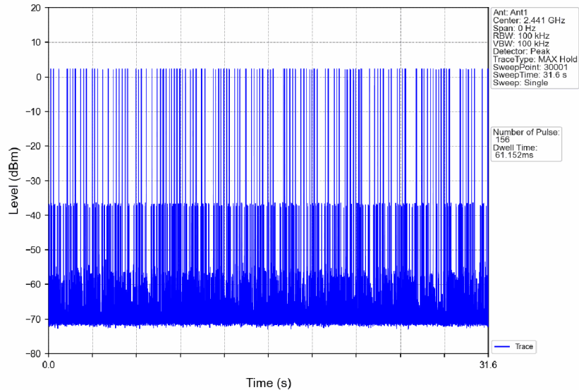
Pi/4DQPSK_2DH3_HOPP_Ant1_NTNV
