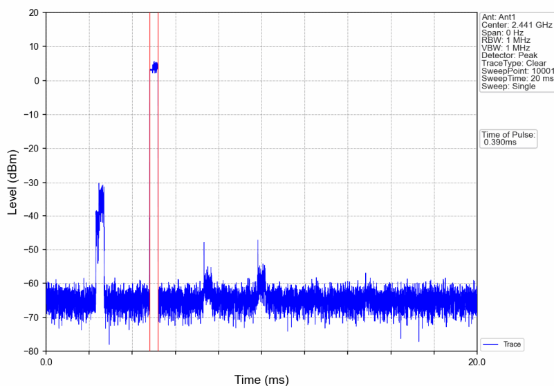
8DPSK_3DH1_HOPP_Ant1_NTNV
