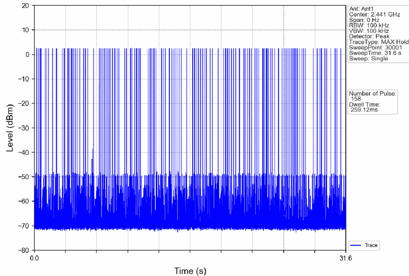
GFSK_DH5_HOPP_Ant1_NTNV
