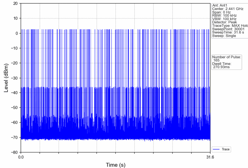
8DPSK_3DH5_HOPP_Ant1_NTNV
