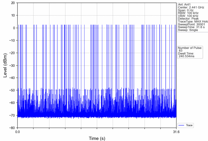
Pi/4DQPSK_2DH1_HOPP_Ant1_NTNV
