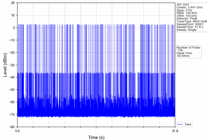
8DPSK_3DH3_HOPP_Ant1_NTNV
