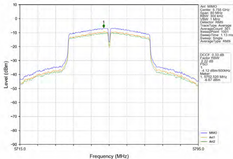
802.11n(HT40)_LCH_5755MHz_MIMO_NTNV
