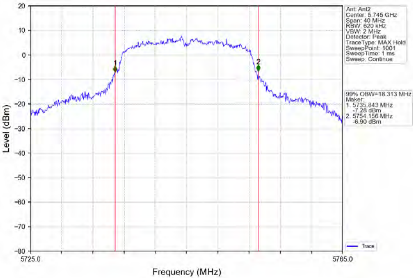
802.11a_LCH_5745MHz_Ant2_NTNV
