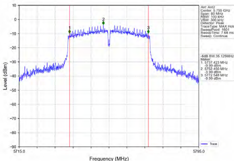
802.11n(HT40)_LCH_5755MHz_Ant2_NTNV
