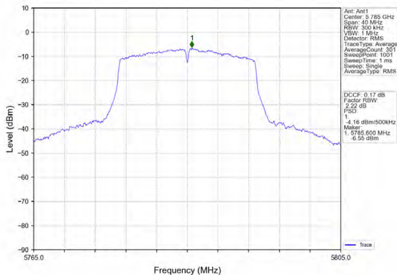
802.11n(HT20)_MCH_5785MHz_Ant1_NTNV
