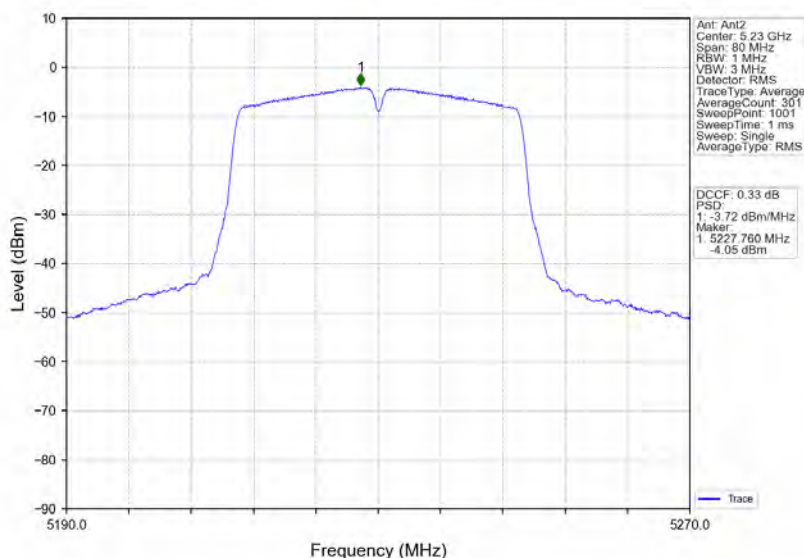
802.11n(HT40)_HCH_5230MHz_Ant2_NTNV
