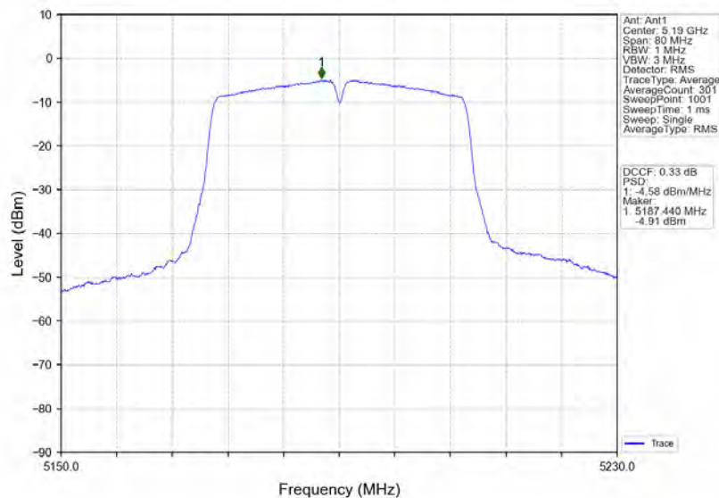
802.11n(HT40)_LCH_5190MHz_Ant1_NTNV
