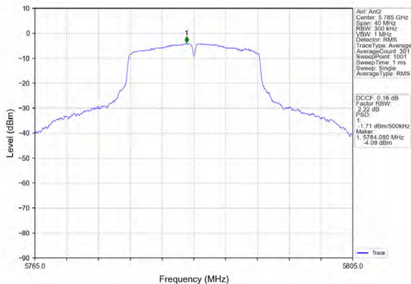
802.11a_MCH_5785MHz_Ant2_NTNV
