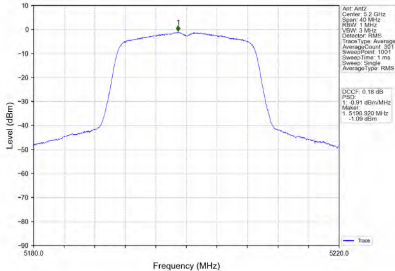
802.11n(HT20)_MCH_5200MHz_MIMO_NTNV
