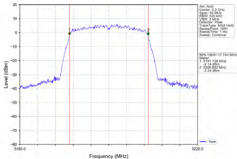
802.11n(HT20)_MCH_5200MHz_Ant2_NTNV
