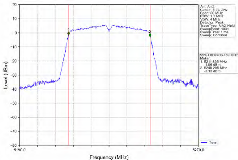
802.11n(HT40)_HCH_5230MHz_Ant2_NTNV
