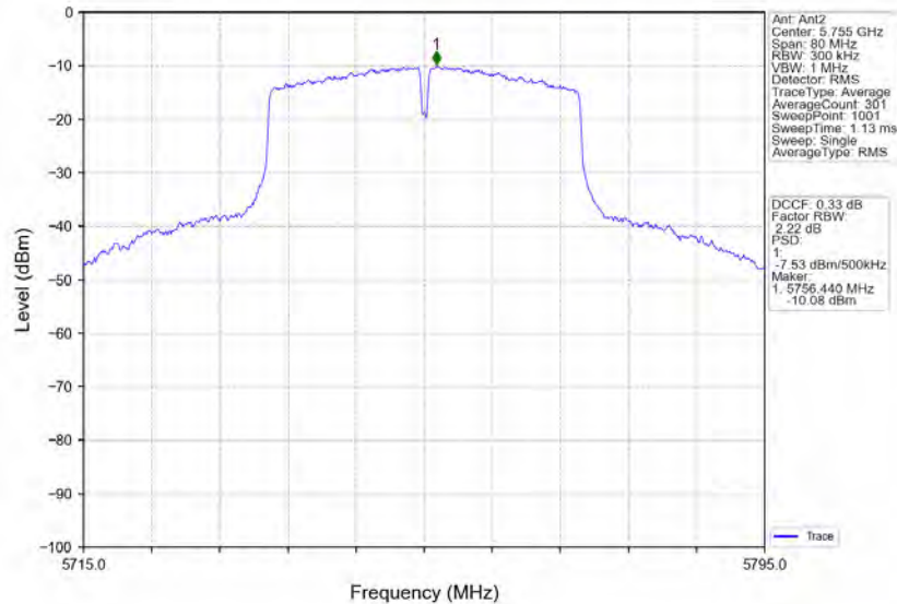
802.11n(HT40)_LCH_5755MHz_MIMO_NTNV
