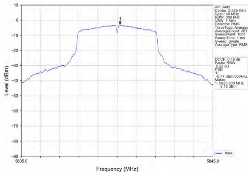
802.11a_HCH_5825MHz_Ant2_NTNV
