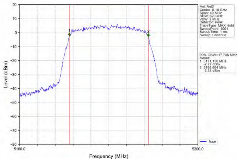
802.11n(HT20)_LCH_5180MHz_Ant2_NTNV
