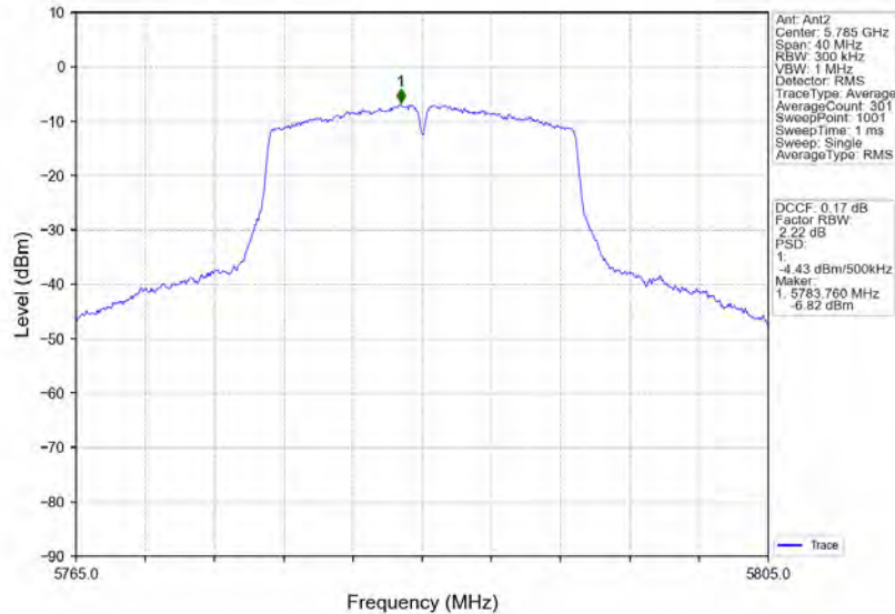
802.11n(HT20)_MCH_5785MHz_MIMO_NTNV
