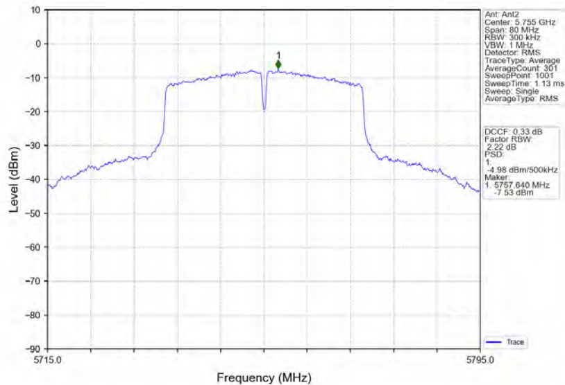
802.11n(HT40)_LCH_5755MHz_MIMO_NTNV
