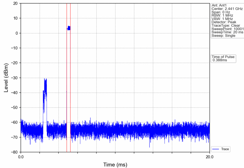
Pi/4DQPSK_2DH1_HOPP_Ant1_NTNV
