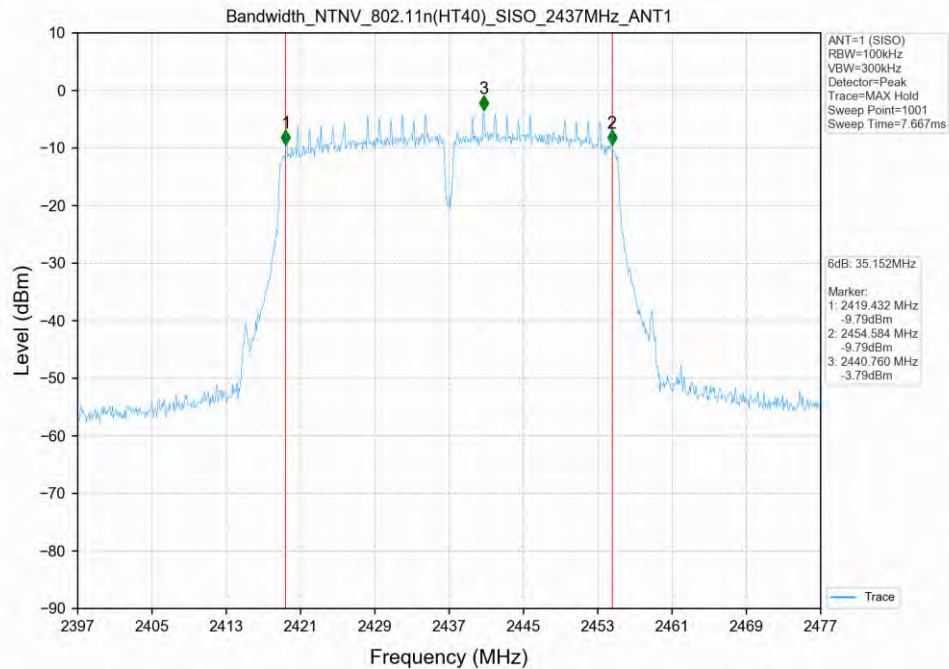
802.11n(HT40)_2437MHz_SISO_ANT1
