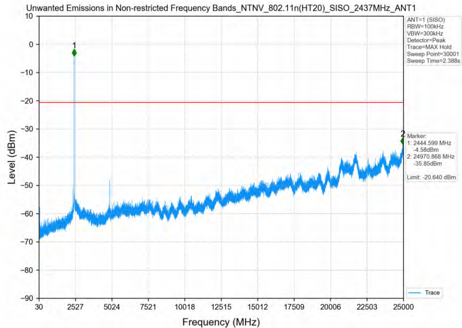
802.11n(HT20)_2437MHz_SISO_ANT1
