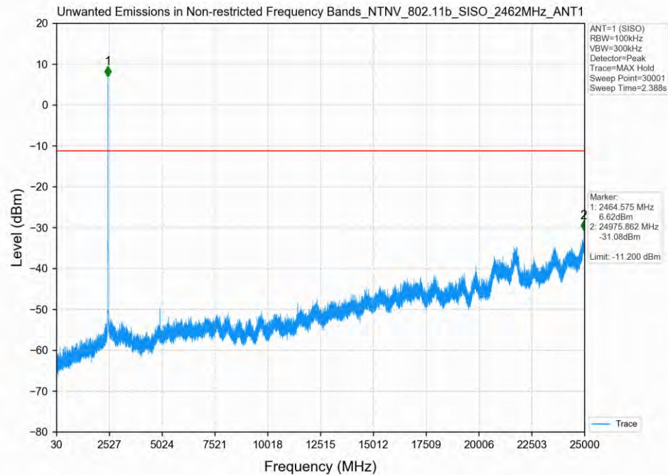
802.11b_2462MHz_SISO_ANT1
