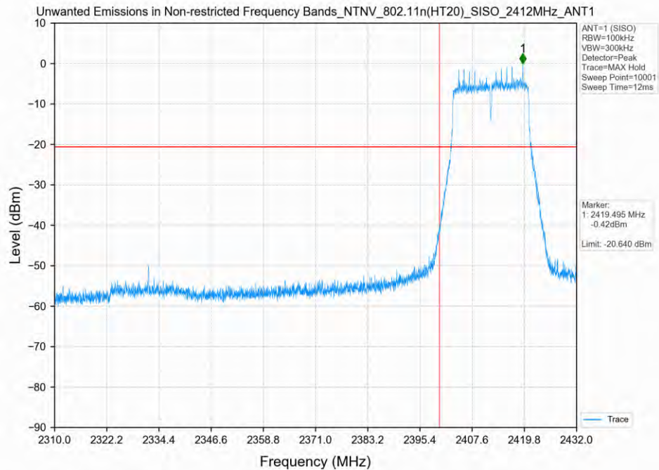
802.11n(HT20)_2412MHz_SISO_ANT1
