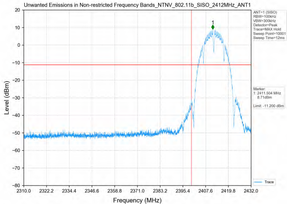
802.11b_2412MHz_SISO_ANT1
