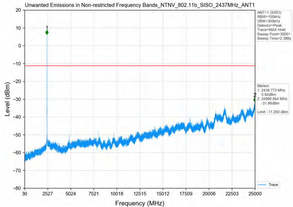
802.11b_2437MHz_SISO_ANT1
