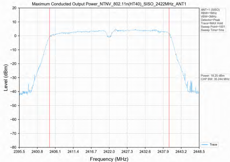
802.11n(HT40)_2422MHz_SISO_ANT1
