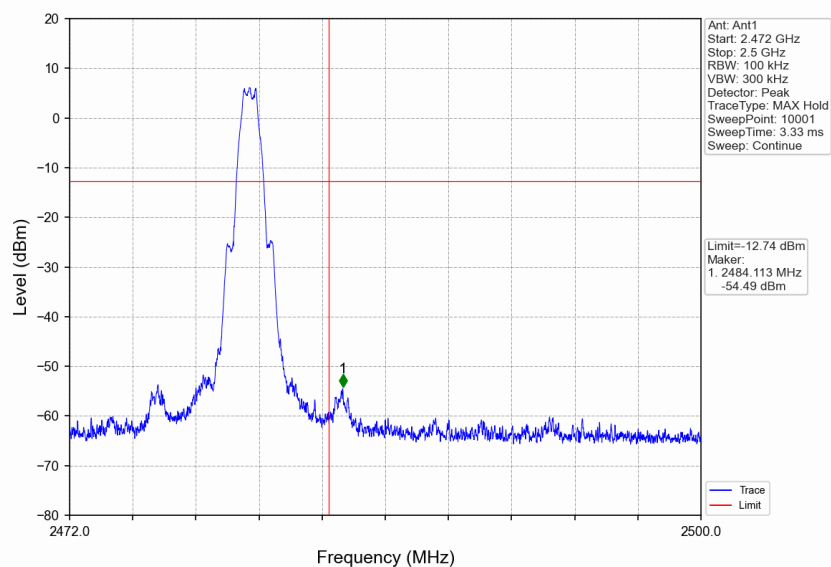
1M_HCH_2480MHz_DataRate=_Ant1_NTNV
