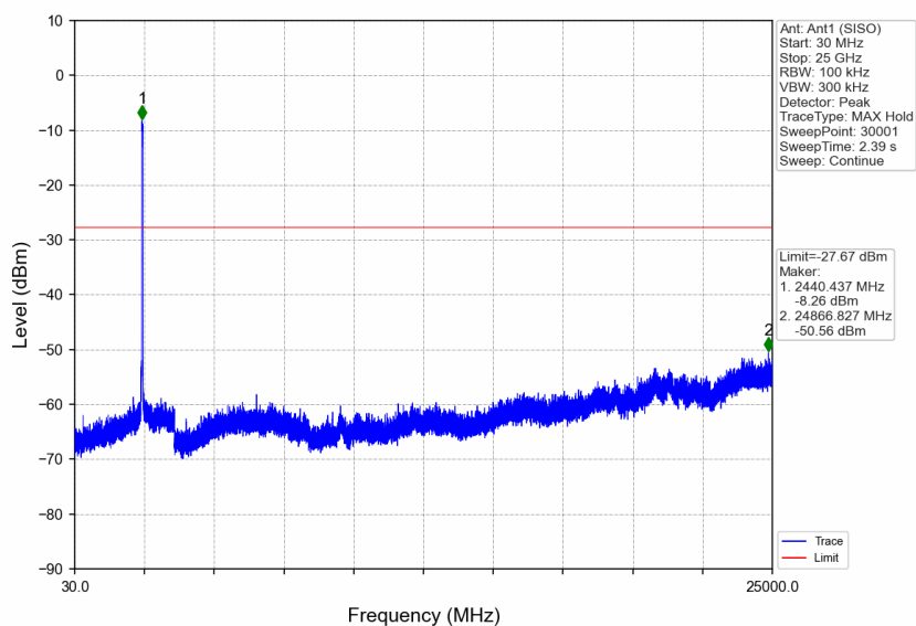
802.11n(HT40)_HCH_2452MHz_Ant1 (SISO)_NTNV
