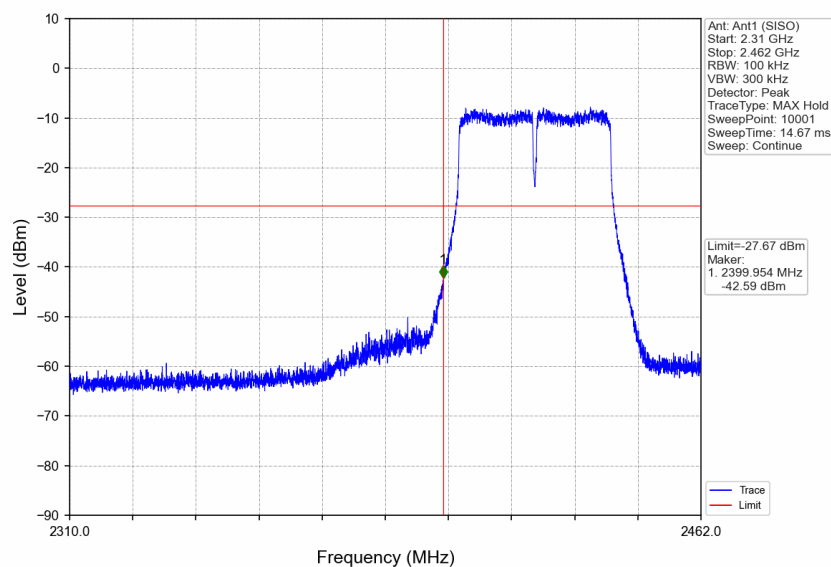
802.11n(HT40)_LCH_2422MHz_Ant1 (SISO)_NTNV
