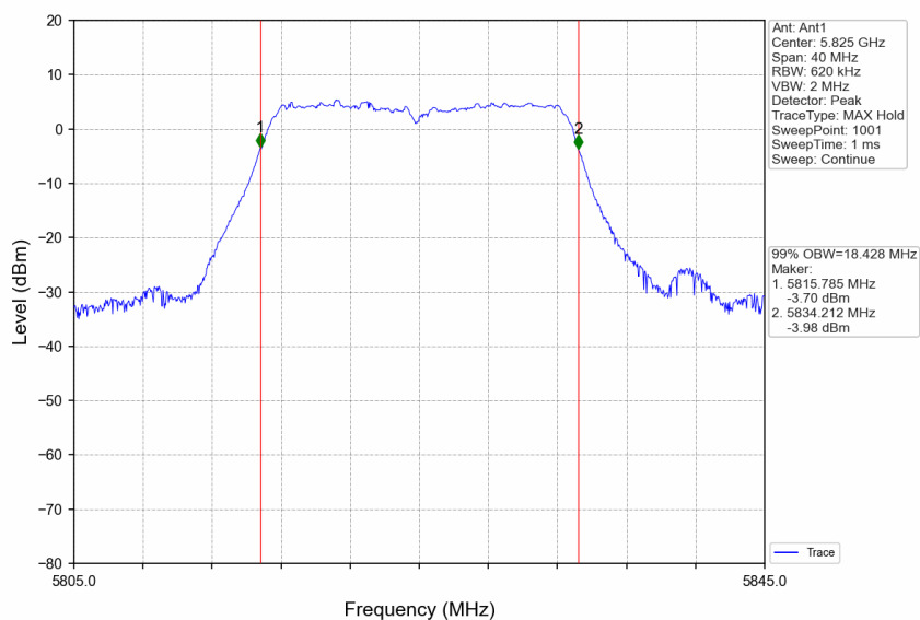
802.11n(HT20)_HCH_5825MHz_Ant1_NTNV
