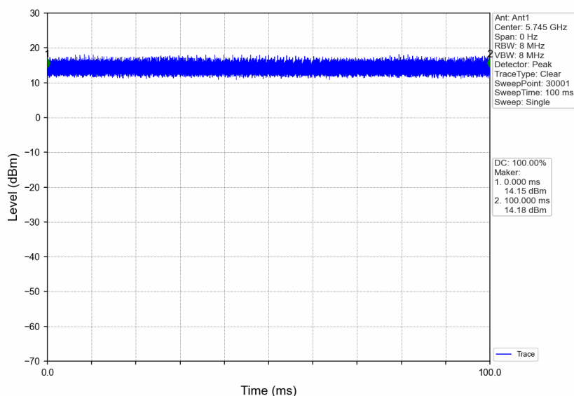
802.11n(HT20)_LCH_5745MHz_Ant1_NTNV
