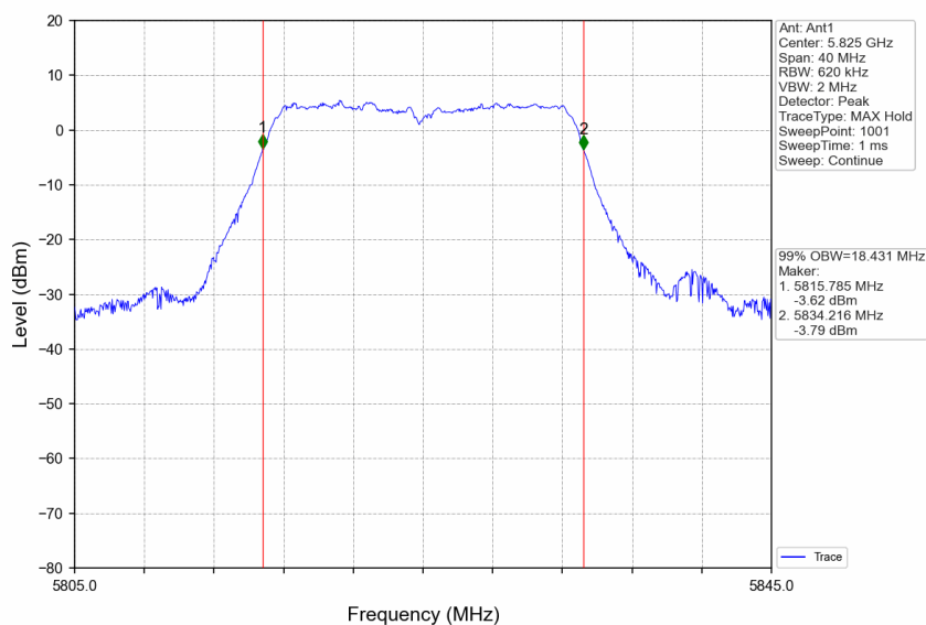
802.11ac(VHT20) HCH_5825MHz_Ant1_NTNV
