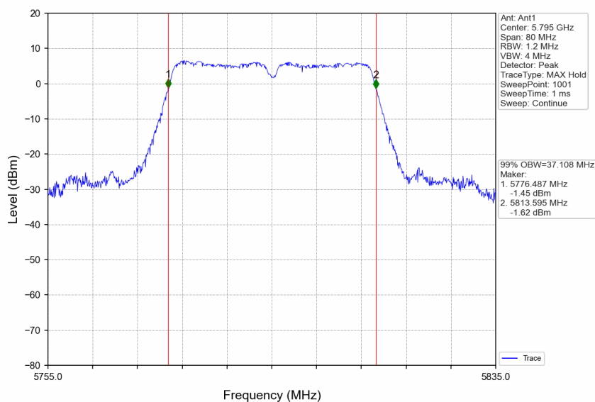
802.11n(HT40)_HCH_5795MHz_Ant1_NTNV
