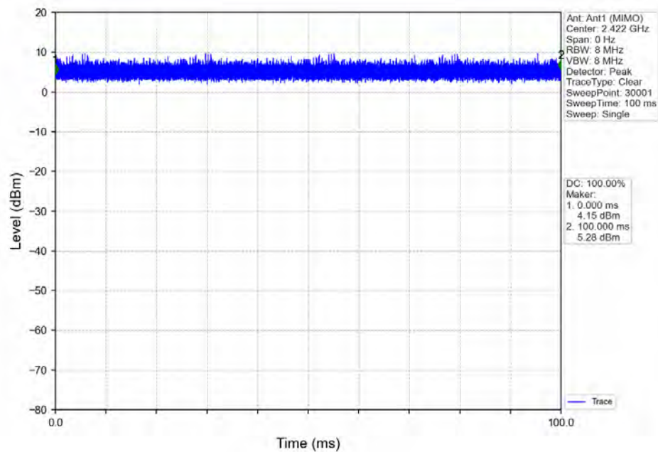
802.11n(HT40)_LCH_2422MHz_Ant1 (MIMO)_NTNV
