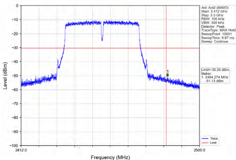
802.11n(HT40)_HCH_2452MHz_Ant2 (MIMO)_NTNV
