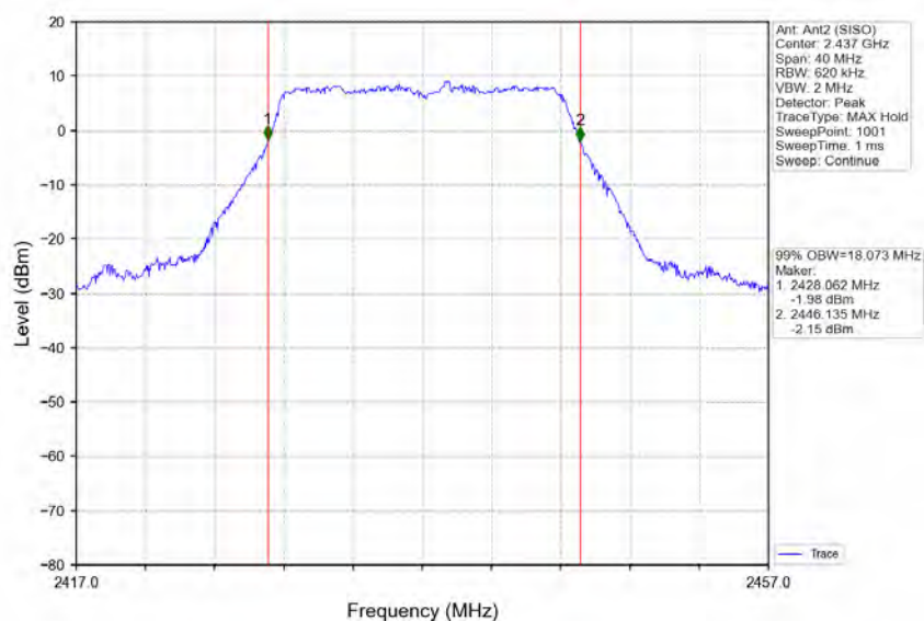
802.11g_MCH_2437MHz_Ant2 (SISO)_NTNV
