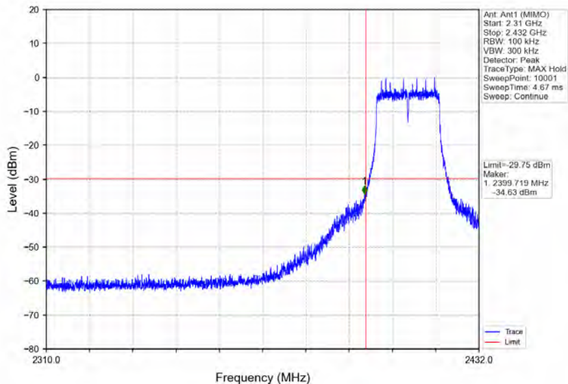
802.11n(HT20)_LCH_2412MHz_Ant1 (MIMO)_NTNV
