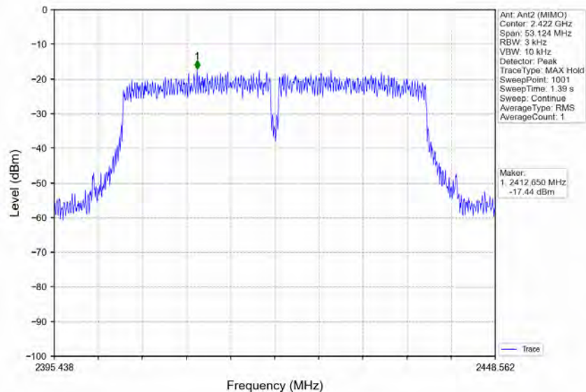
802.11n(HT40) LCH_2422MHz_MIMO_NTNV
