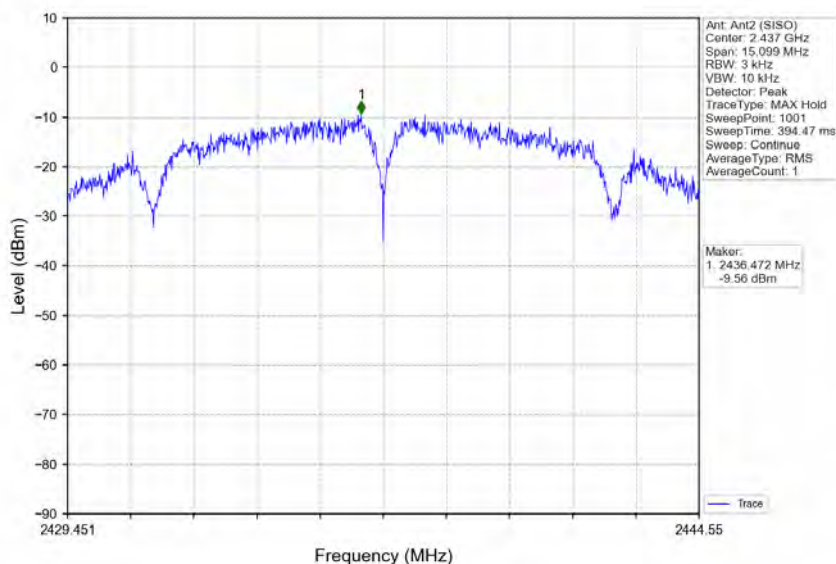
802.11b_MCH_2437MHz_Ant2 (SISO)_NTNV
