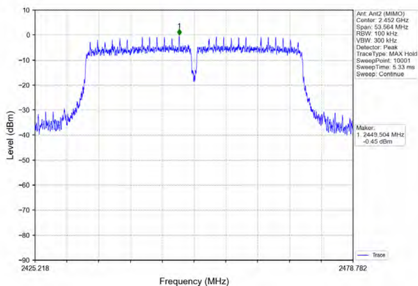
802.11n(HT40)_HCH_2452MHz_Ant2 (MIMO)_NTNV
