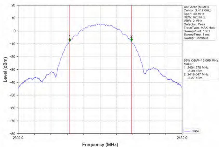
802.11n(HT20)_LCH_2412MHz_Ant2 (MIMO)_NTNV
