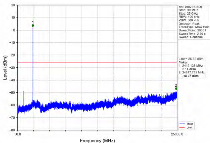
802.11b_LCH_2412MHz_Ant2 (SISO)_NTNV
