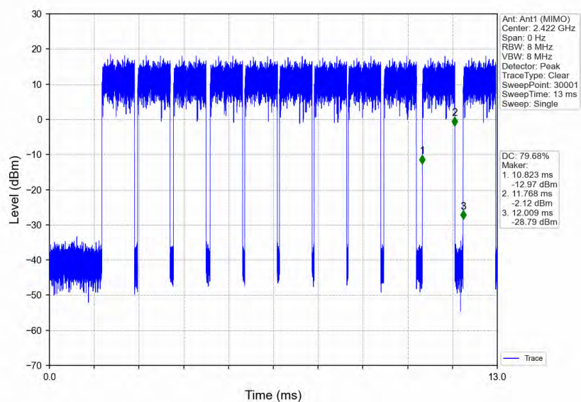
802.11n(HT40)_LCH_2422MHz_Ant1 (MIMO)_NTNV
