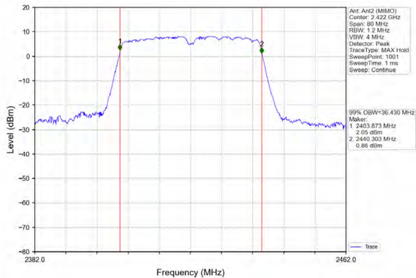
802.11n(HT40)_LCH_2422MHz_Ant2 (MIMO)_NTNV
