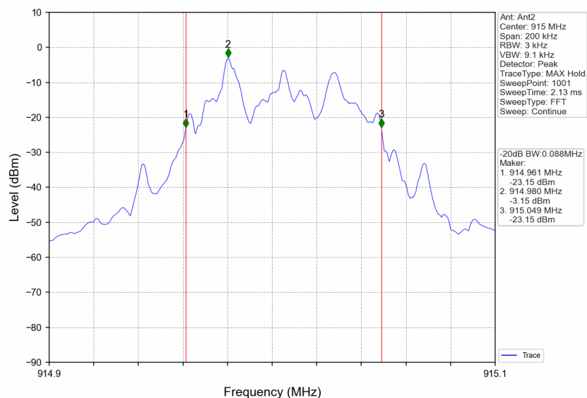
FSK_MCH_915MHz_Ant2_NTNV
