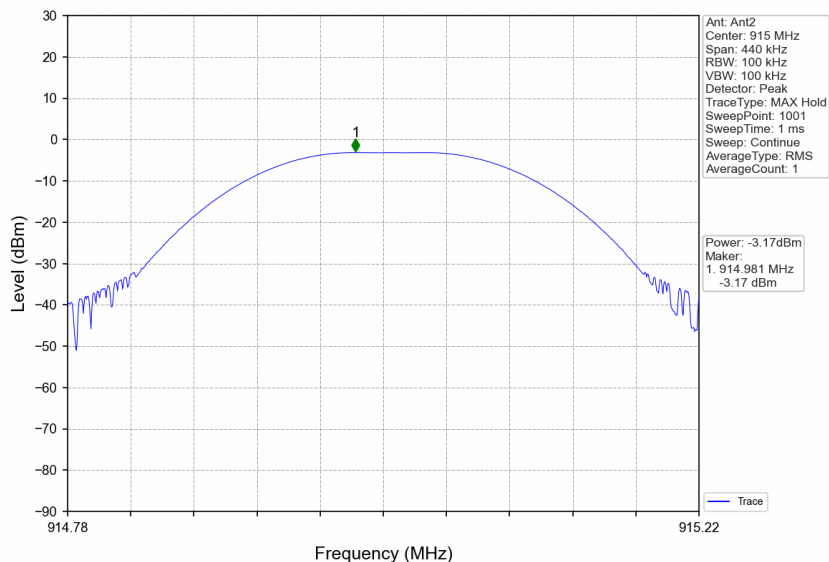
FSK_MCH_915MHz_Ant2_NTNV
