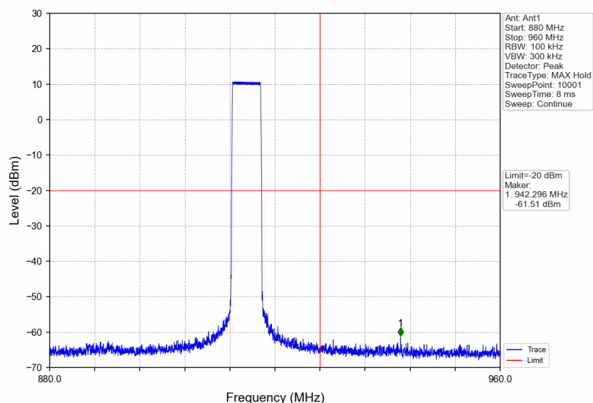
FSK_HOPP_Ant1_NTNV
