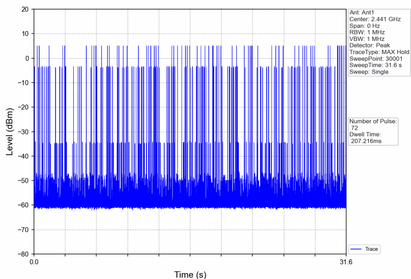
GFSK_DH5_HOPP_Ant1_NTNV
