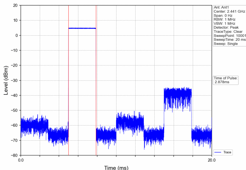
GFSK_DH5_HOPP_Ant1_NTNV
