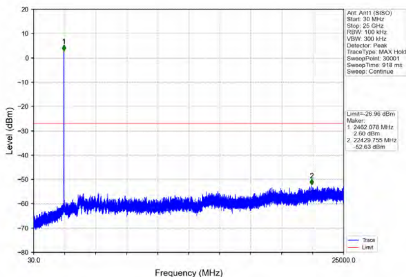
802.11b_HCH_2462MHz_Ant1 (SISO)_NTN
