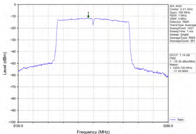
802.11ac(VHT80)_MCH_5210MHz_Ant2_NTNV
