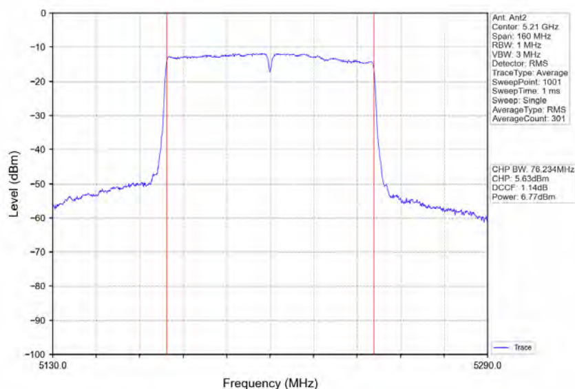
802.11ac(VHT80)_MCH_5210MHz_Ant2_NTNV
