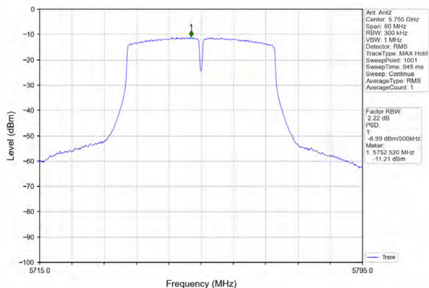
802.11n(HT40) LCH 5755MHz MIMO NTV
