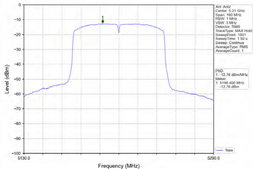
802.11ac(VHT80)_MCH_5210MHz_Ant2_NTNV
