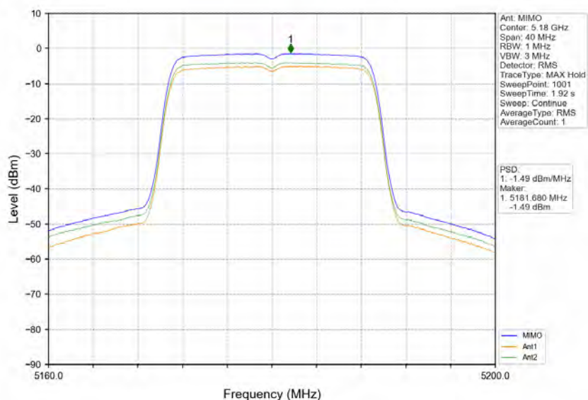
802.11ac(VHT20) LCH 5180MHz MIMO NTN
