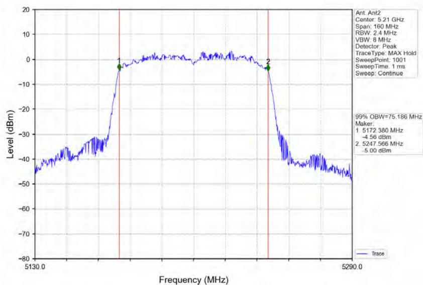
802.11ac(VHT80)_MCH_5210MHz_Ant2_NTNV
