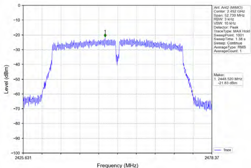
802.11n(HT40) HCH 2452MHz MIMO NTNV
