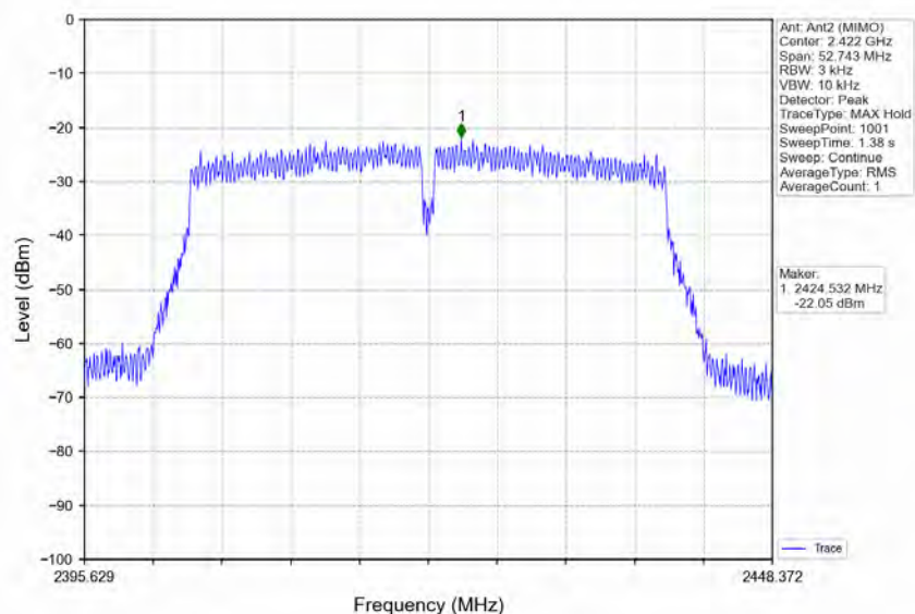
802.11n(HT40) LCH 2422MHz MIMO NTNV
