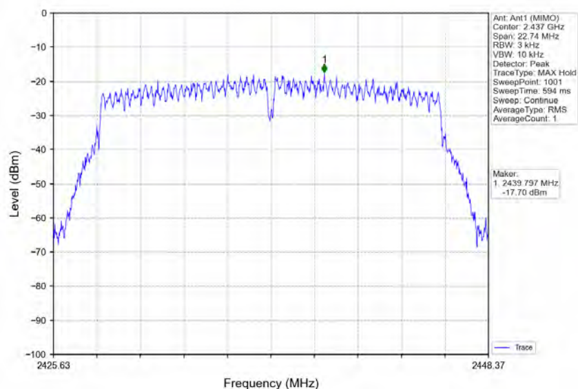
802.11n(HT20)_MCH_2437MHz_Ant1 (MIMO)_NTNV
