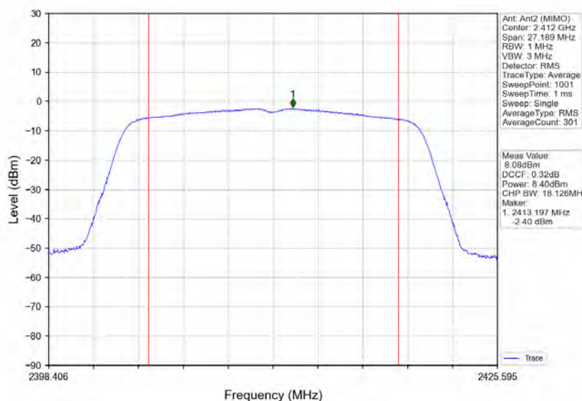
802.11n(HT20) LCH 2412MHz Ant2 (MIMO) NTNV
