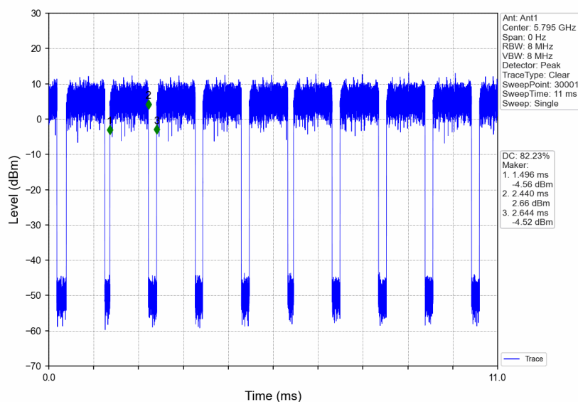
802.11n(HT40)_HCH_5795MHz_Ant1_NTNV
