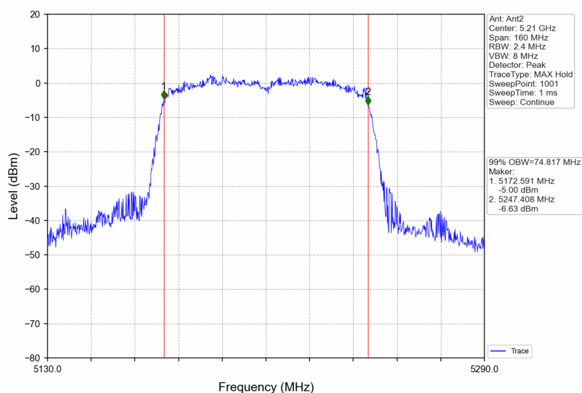
802.11ac(VHT80)_MCH_5210MHz_Ant2_NTNV
